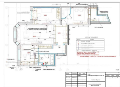
План размещения розеточных групп с привязками
