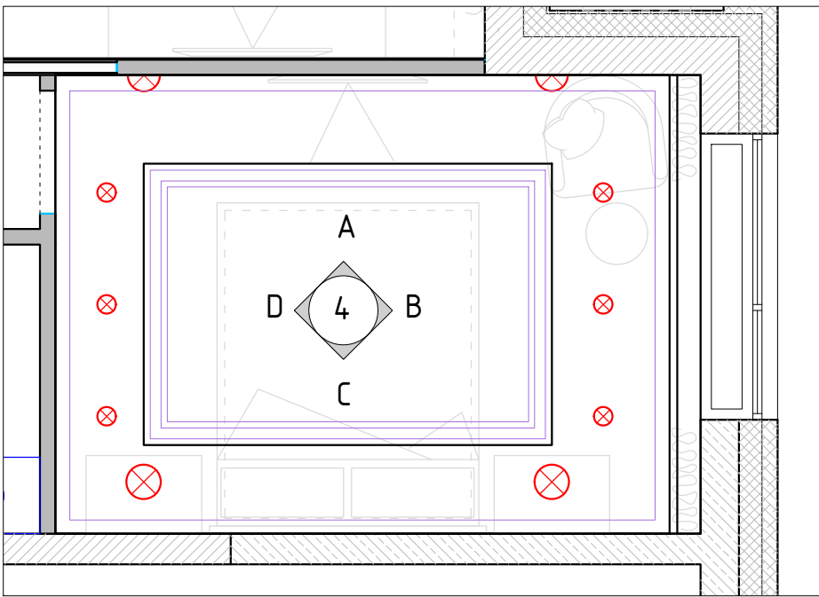
План света и потолка
