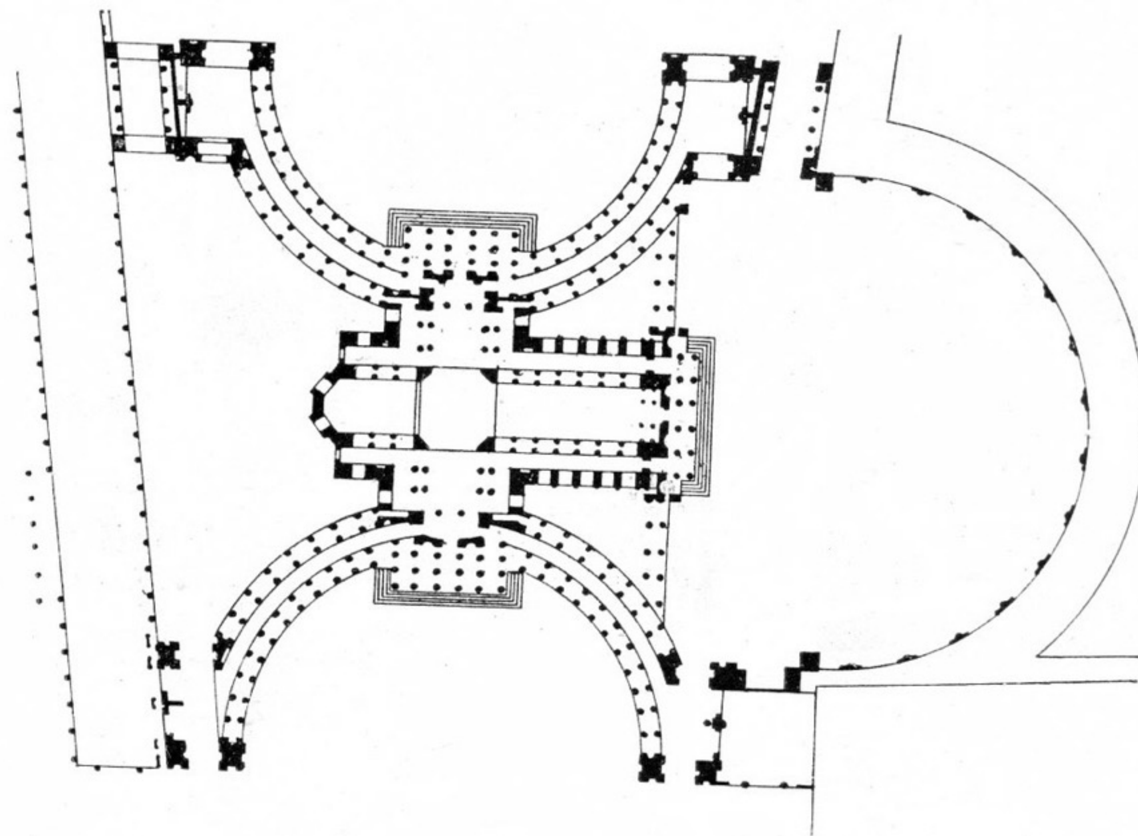
А. Н. Воронихин. Казанский собор в Ленинграде. Проект 1810 г. План
