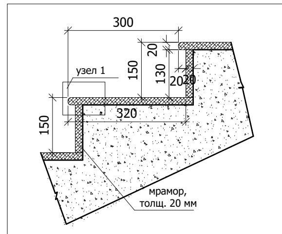
Лестница.Фрагмент. М 1:10
