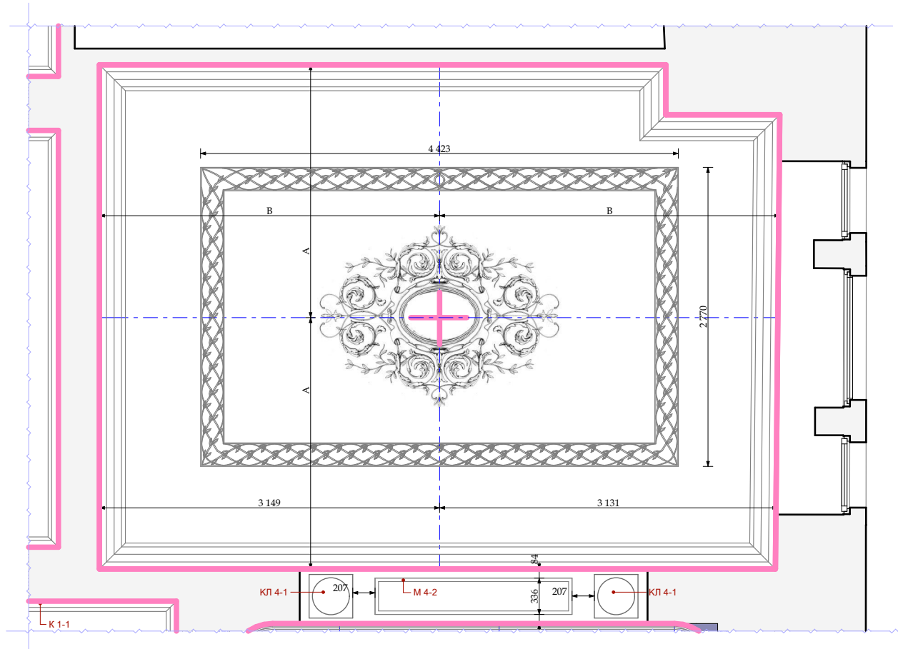
План потолка
