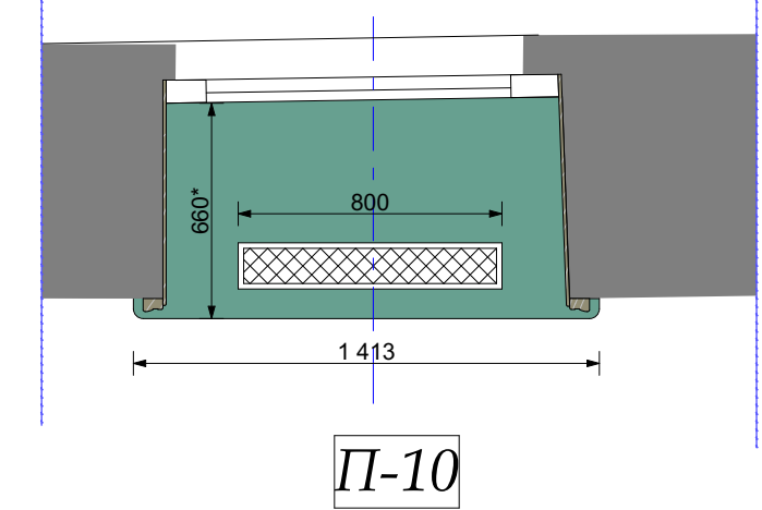
Гардеробная №17
