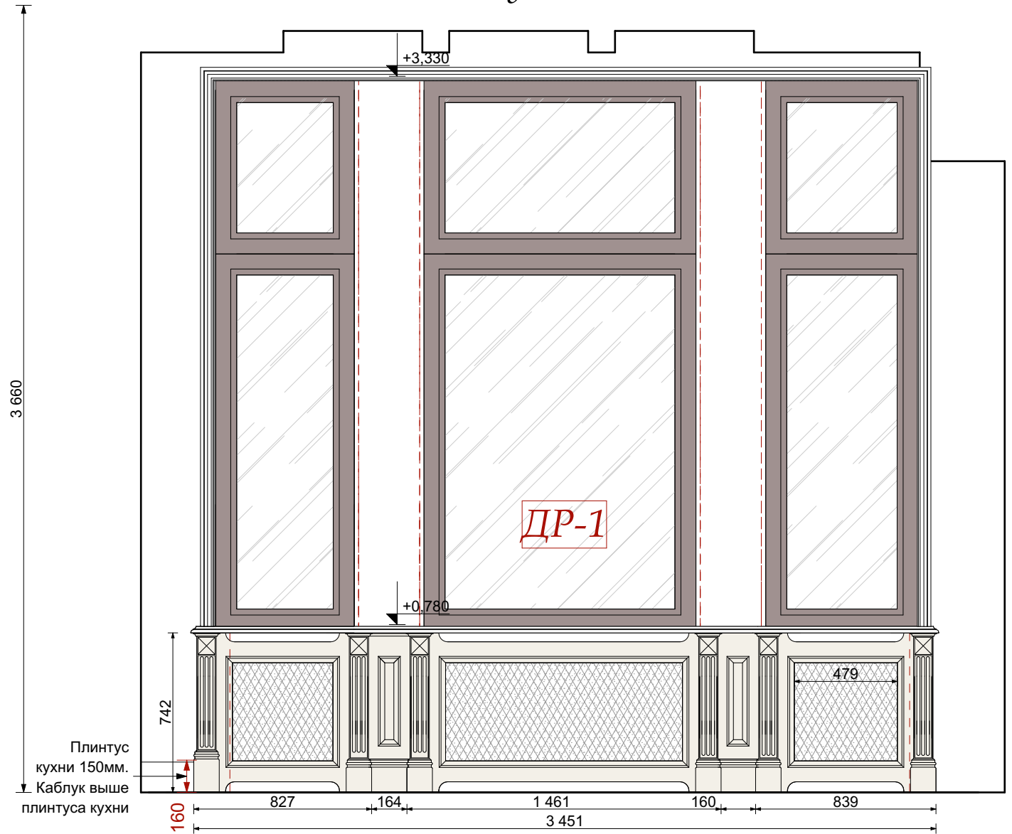
Кухня №6
