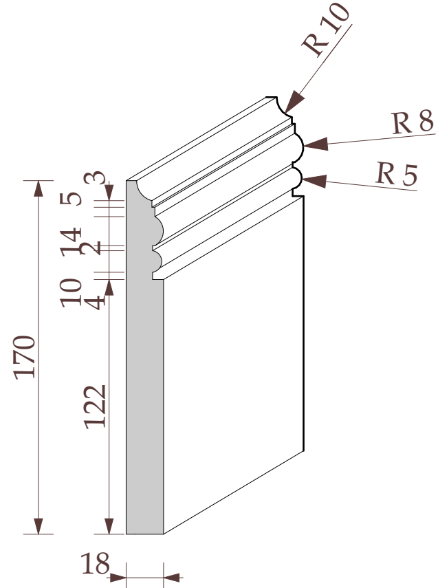
ПЛИНТУС ТИП 2
