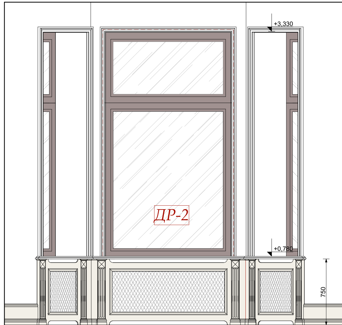
Столовая №5
