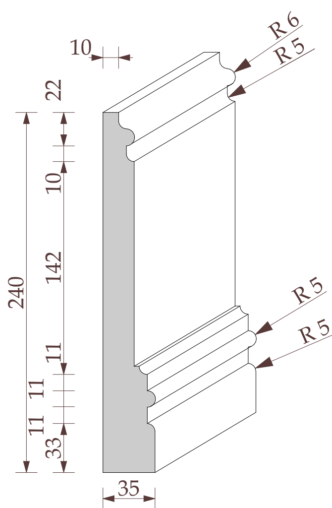
ПЛИНТУС ТИП 1
