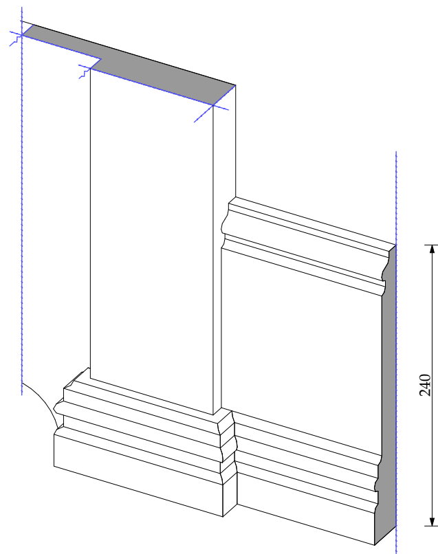
плинтус Тип 2
