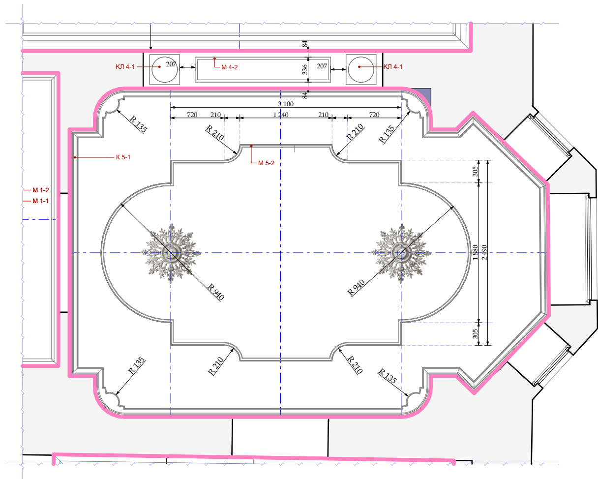
План потолка
