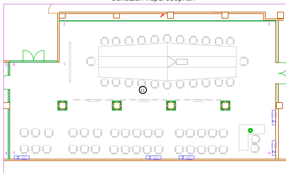
План. 1:150 Большая переговорная
