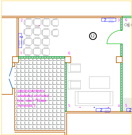
План М 1:150 Комната ожидания/ кладовая
