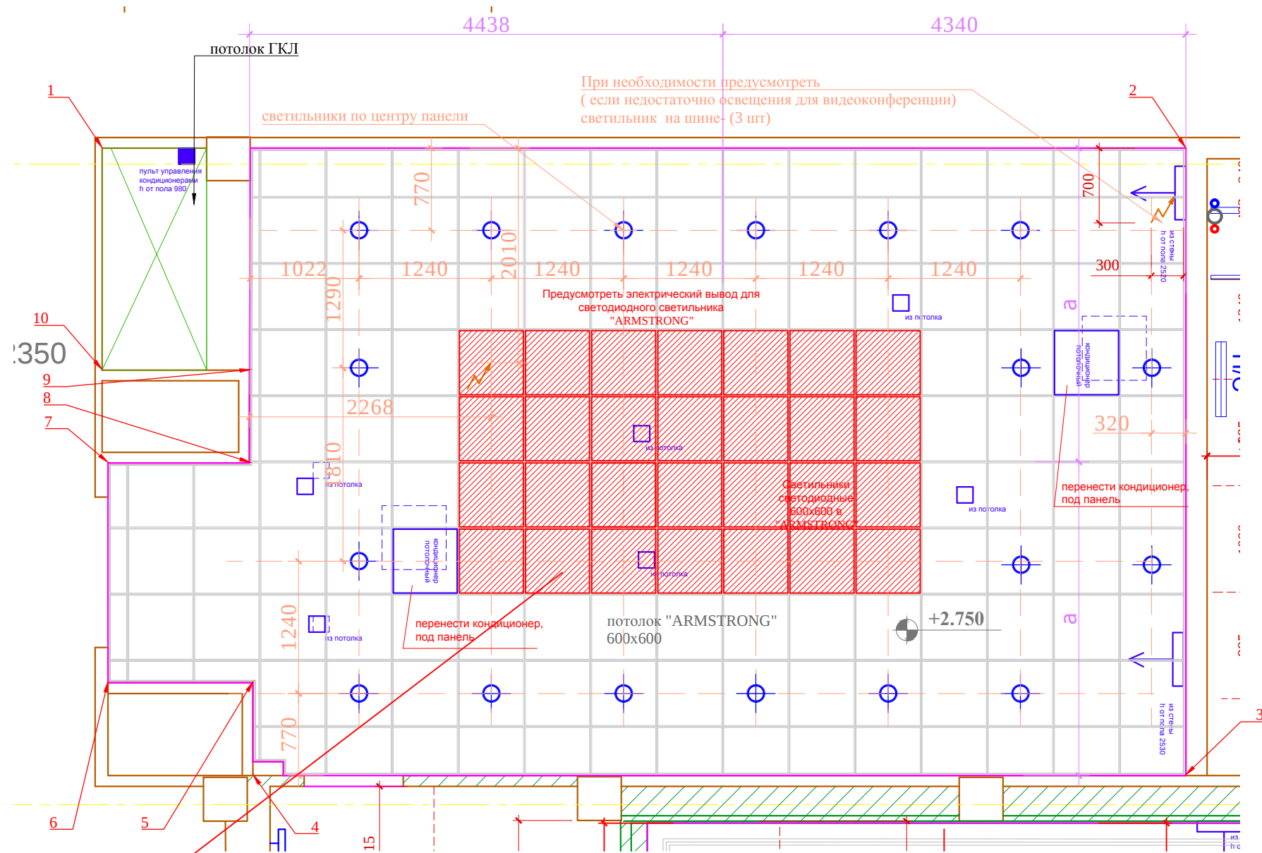
План потолка с расстановкой осветительного оборудования. М1:50
