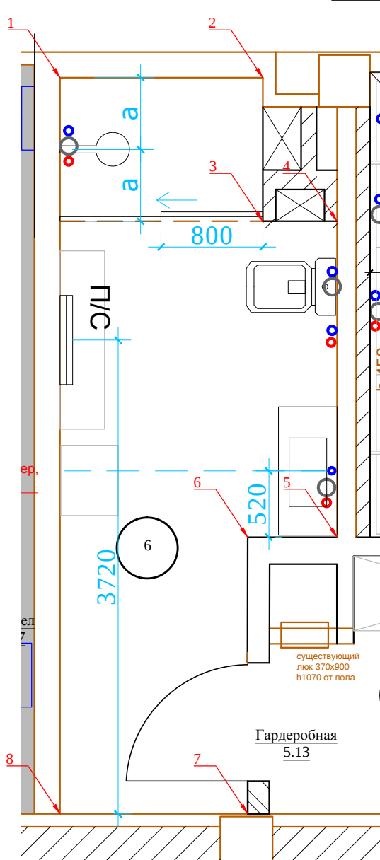
План сантехники. М1:40
