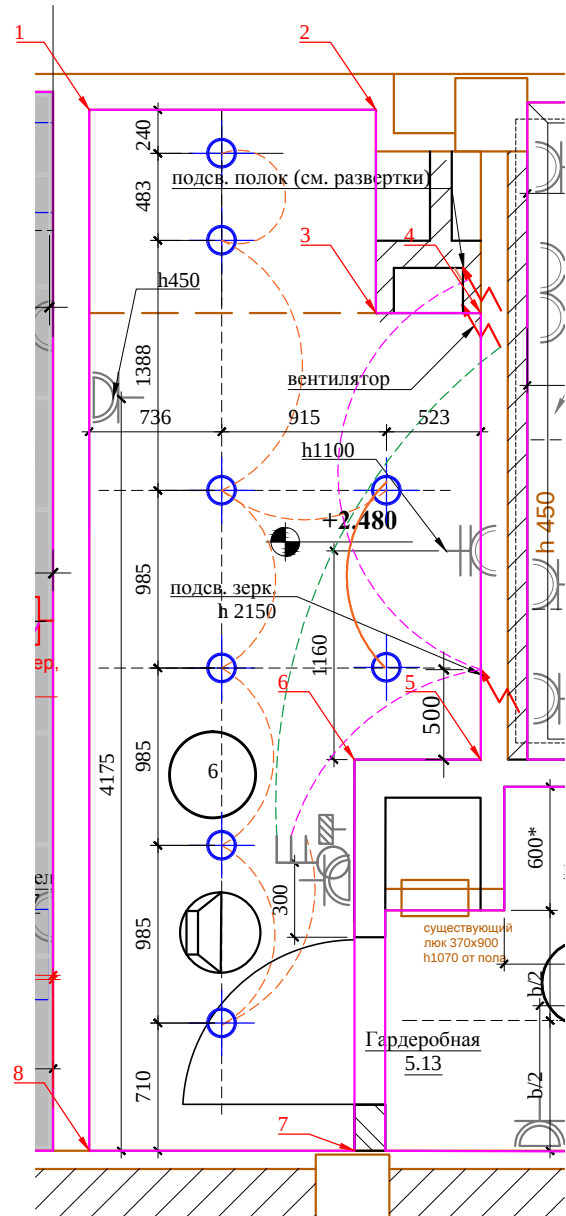
План электрики. М1:40
