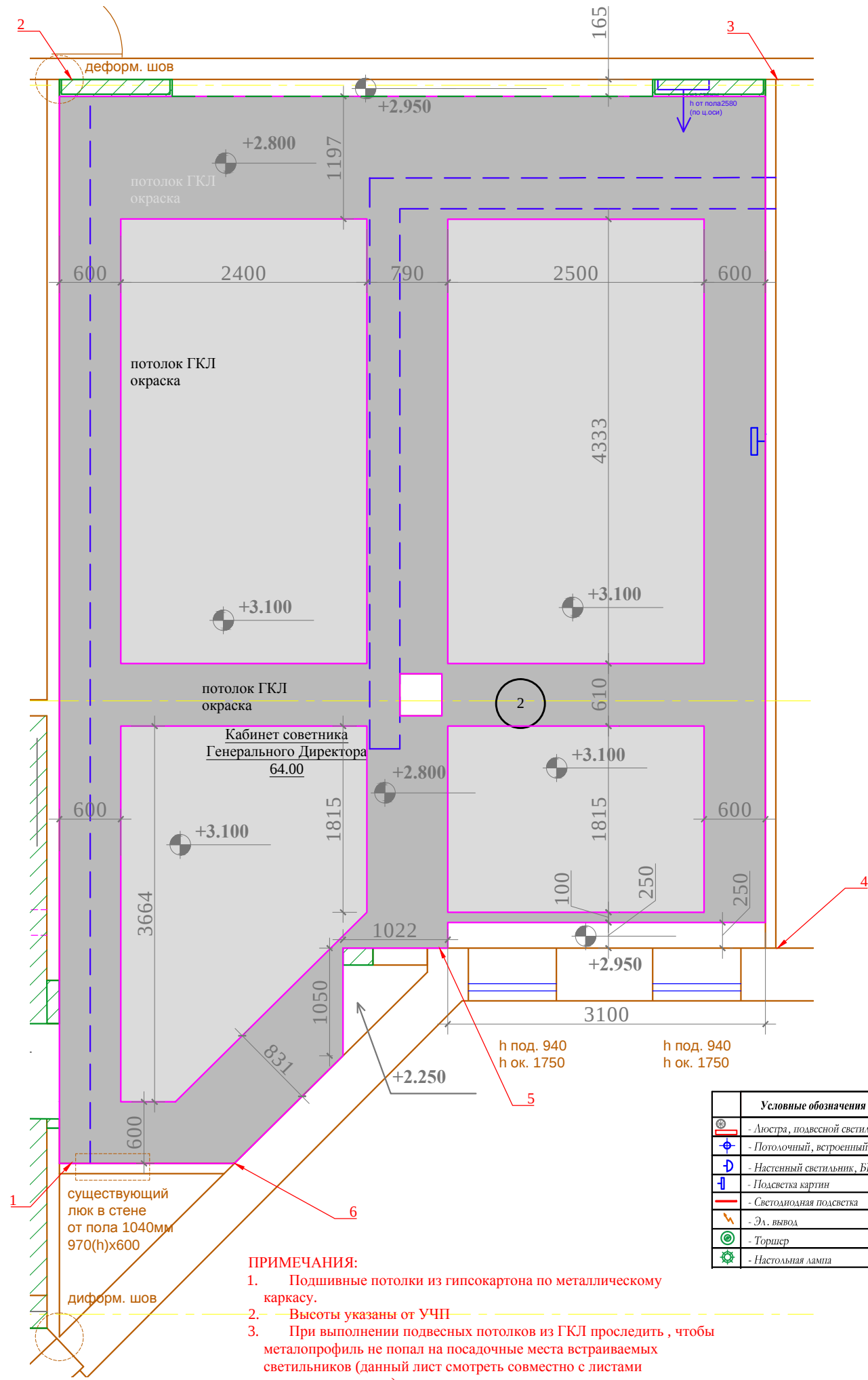
План потолка.
