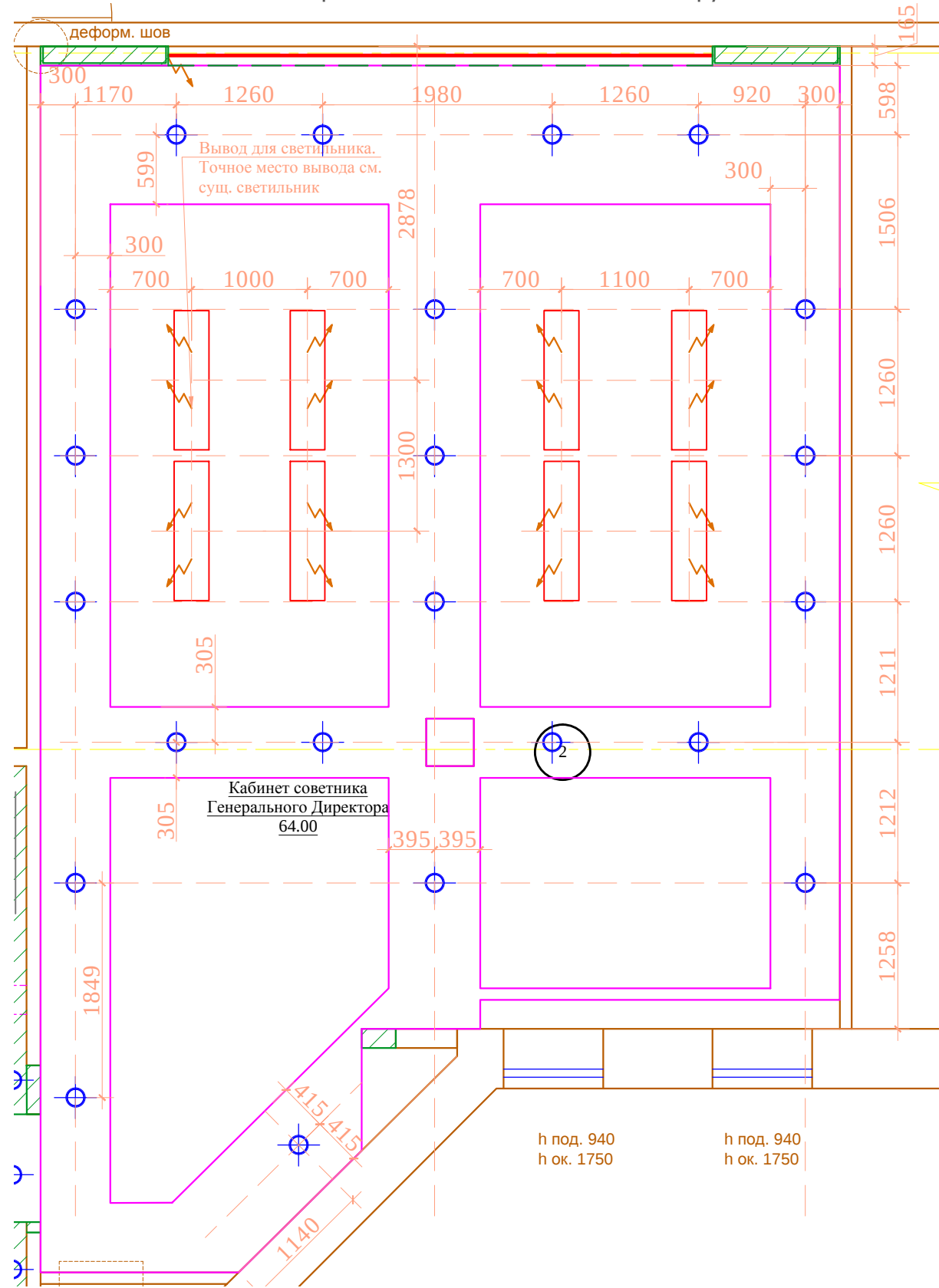
План потолков с расстановкой осветительного оборудования.
