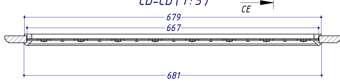
CD-CD (1:5)
