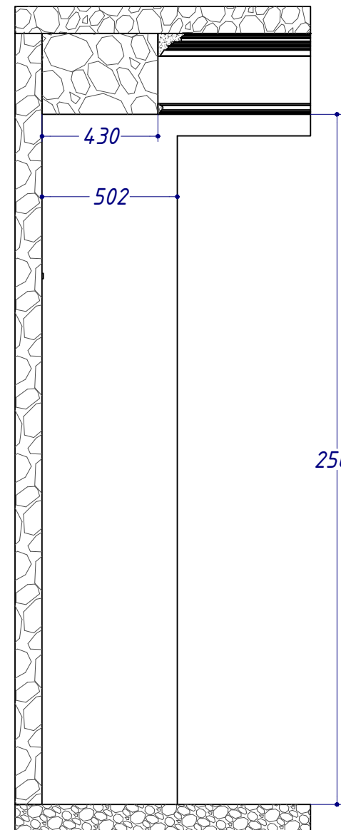
А-А (1:20)
