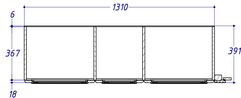
AA-AA (1:15)
