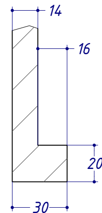
AU (1:2)
