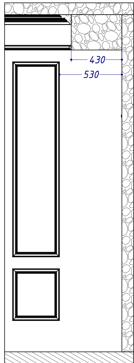
В-В (1:20)
