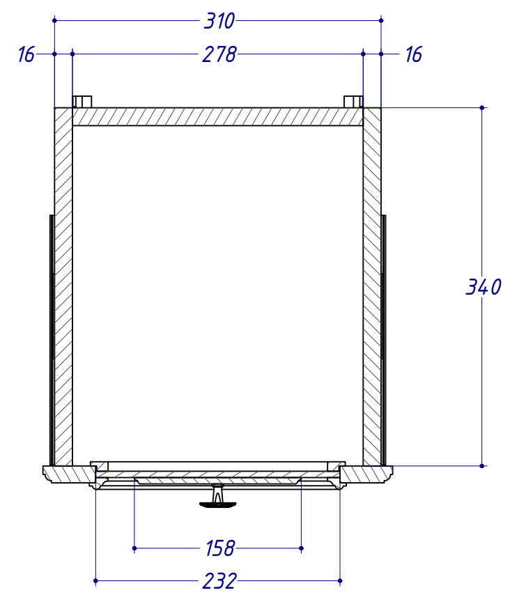
BH-BH (1:5)
