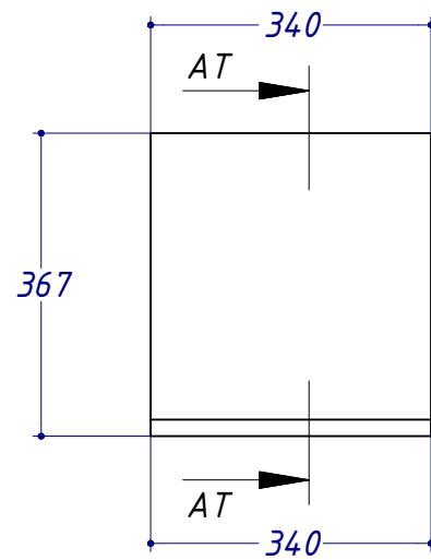
ВИД 10 (1:10)
