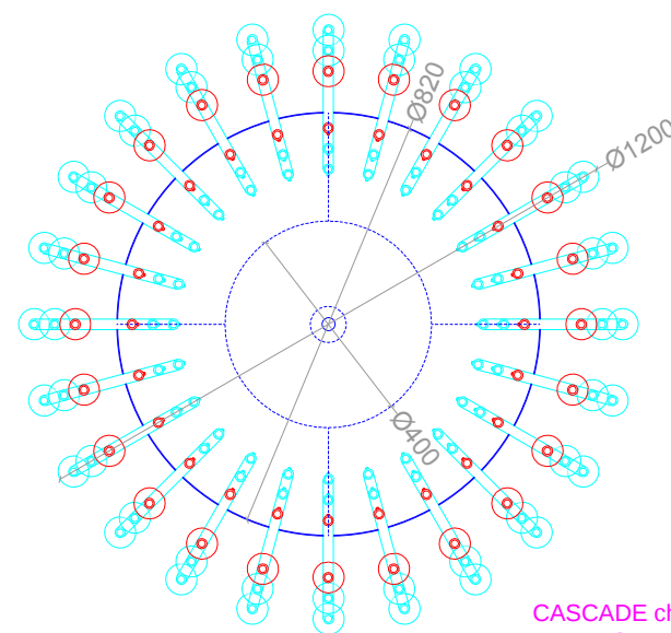
PIANTA
