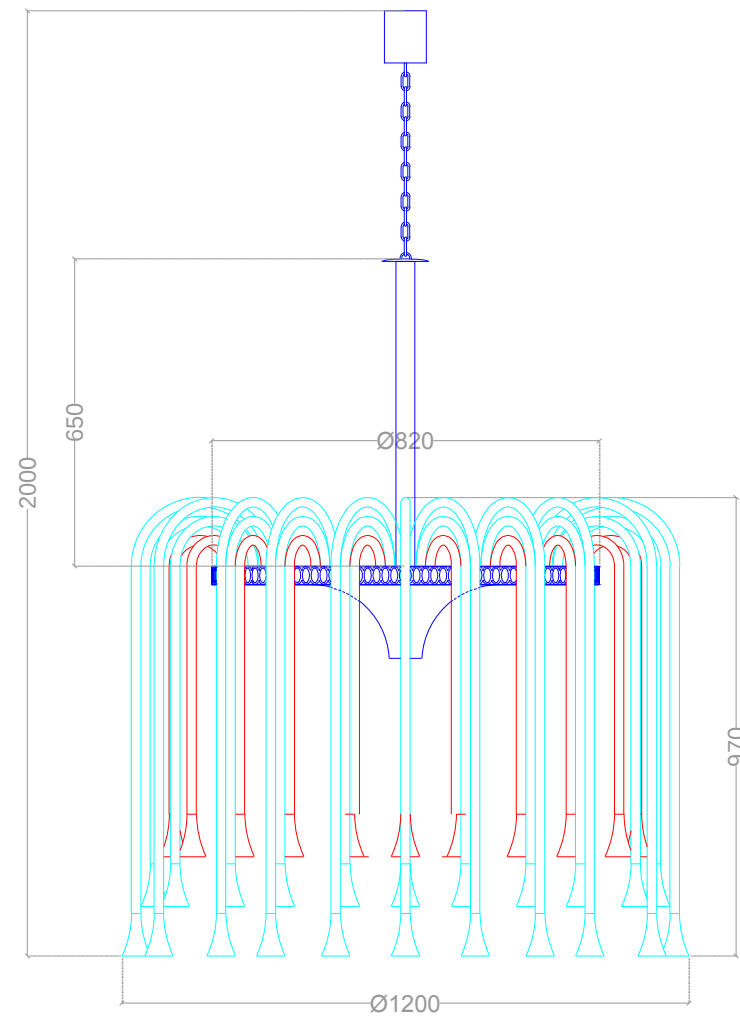
VISTA FRONTALE
