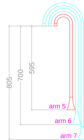
VISTA LATERALE ELEMENTI
