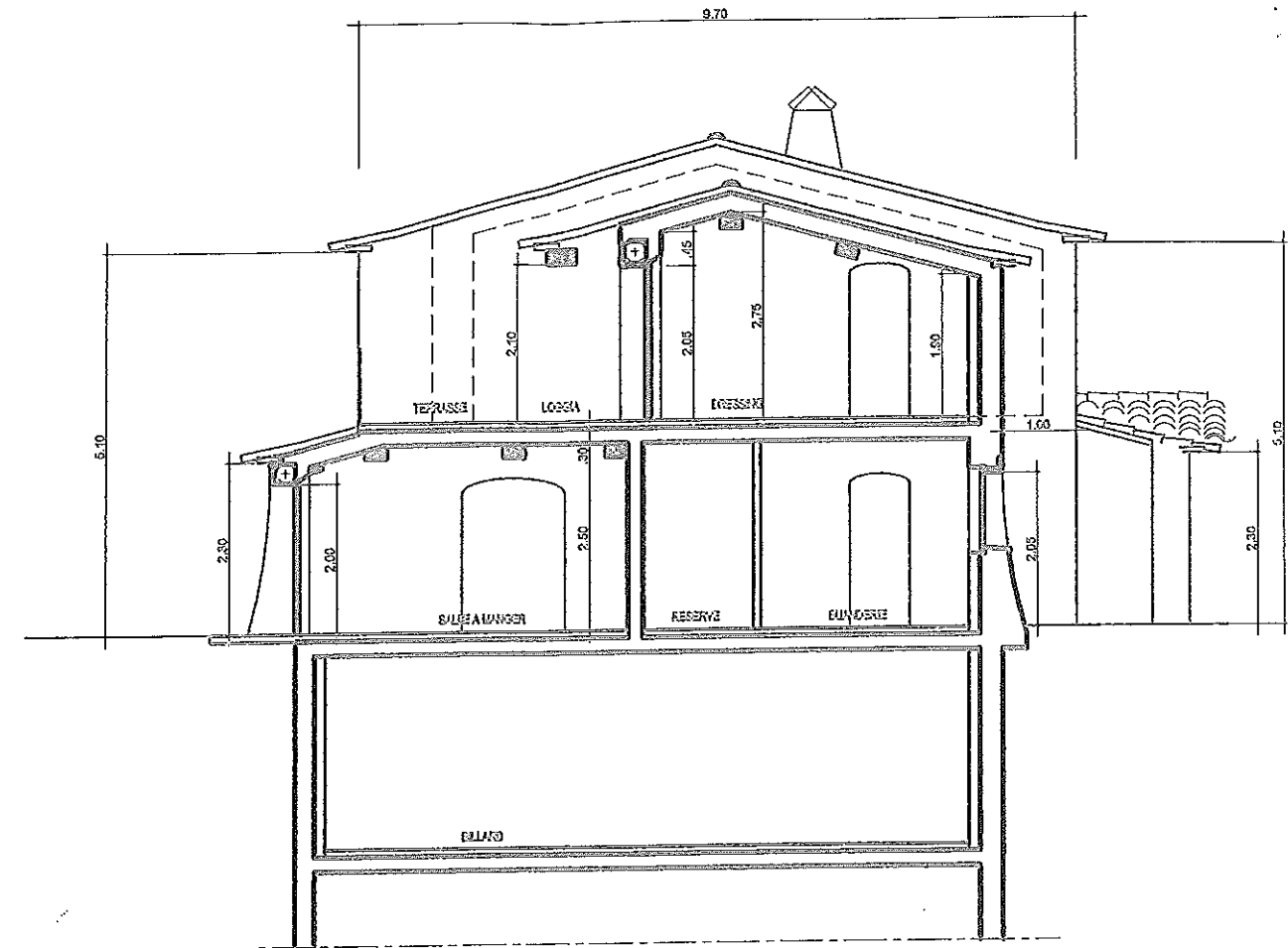
COUPE B - B
