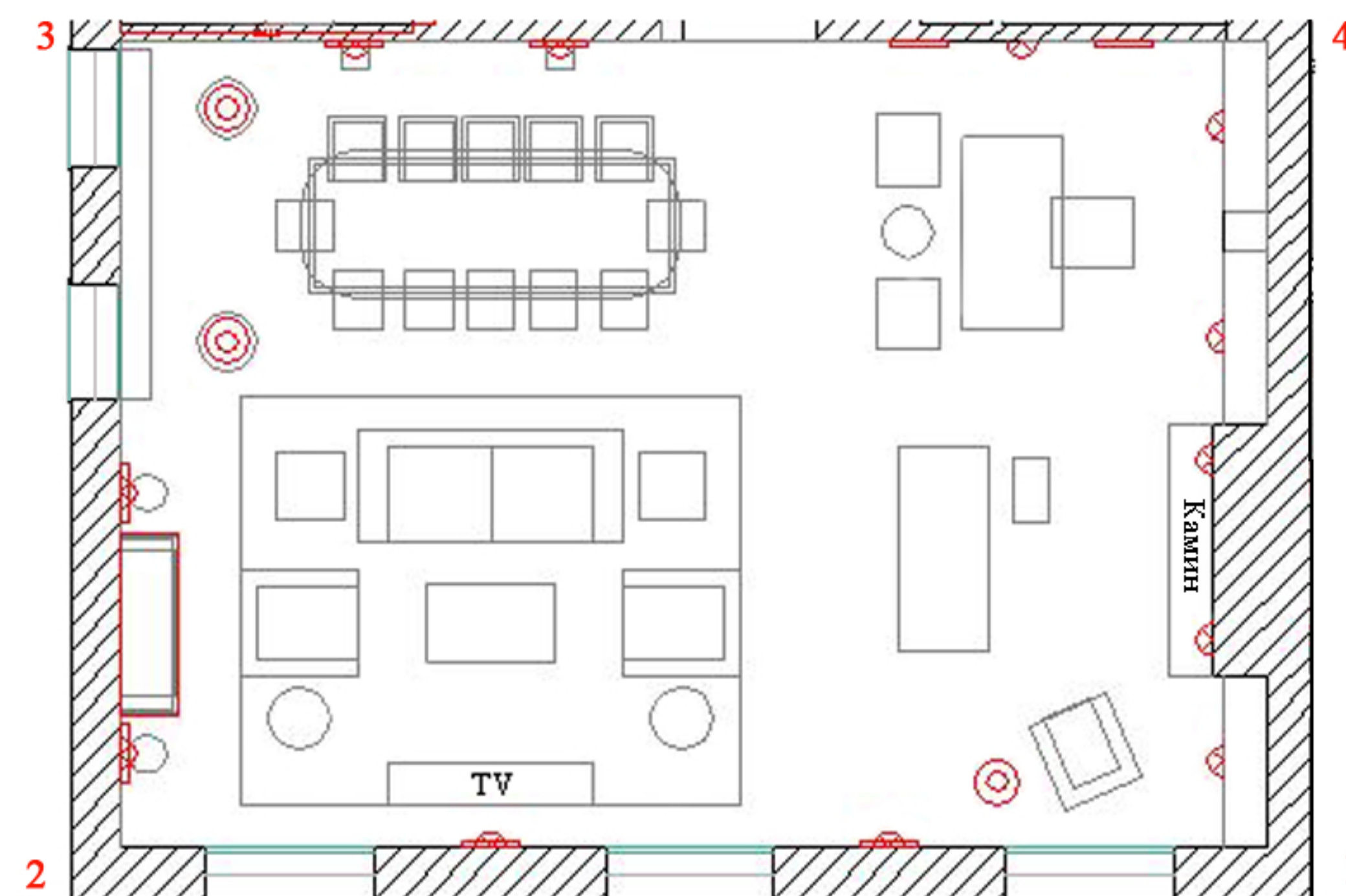
План Гостиной-Столовой.
