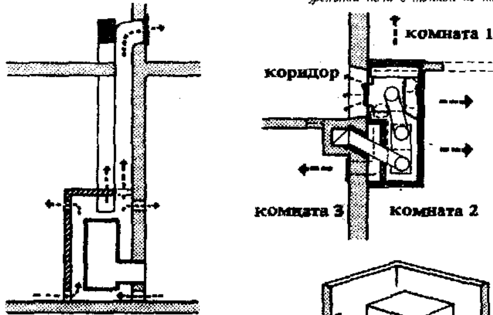
2. Центральное отопление многоэтажного дома от кафельной печи
