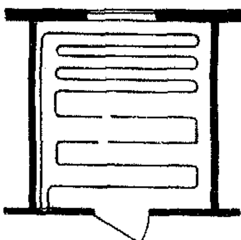
8. Число труб регистра лучистого отопления увеличивается у наружных стен
