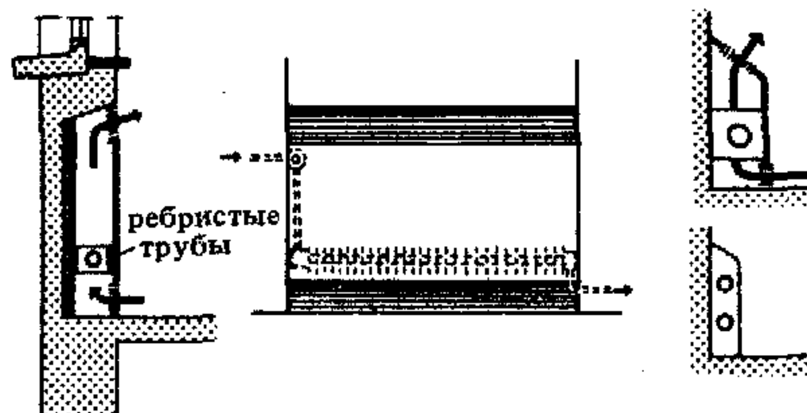
5. Конвекторы из стальных или медных ребристых труб с передней стенкой в виде щитуса
