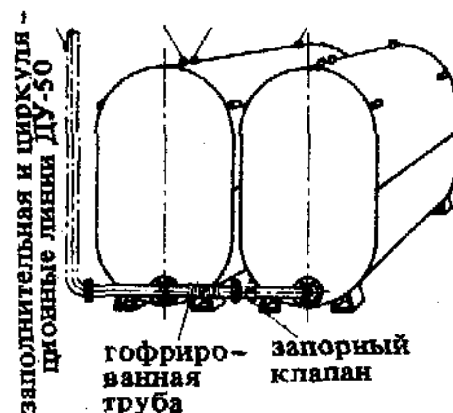
4. Групповые цистерны для жидкого топлива, устанавливаемые в подвале
