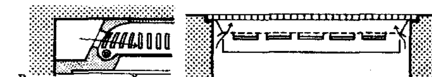
Вентиляционный канал с углублением для установки источника света и доступная приточная или вытяжная решетка с кожухом для защиты от пыли
