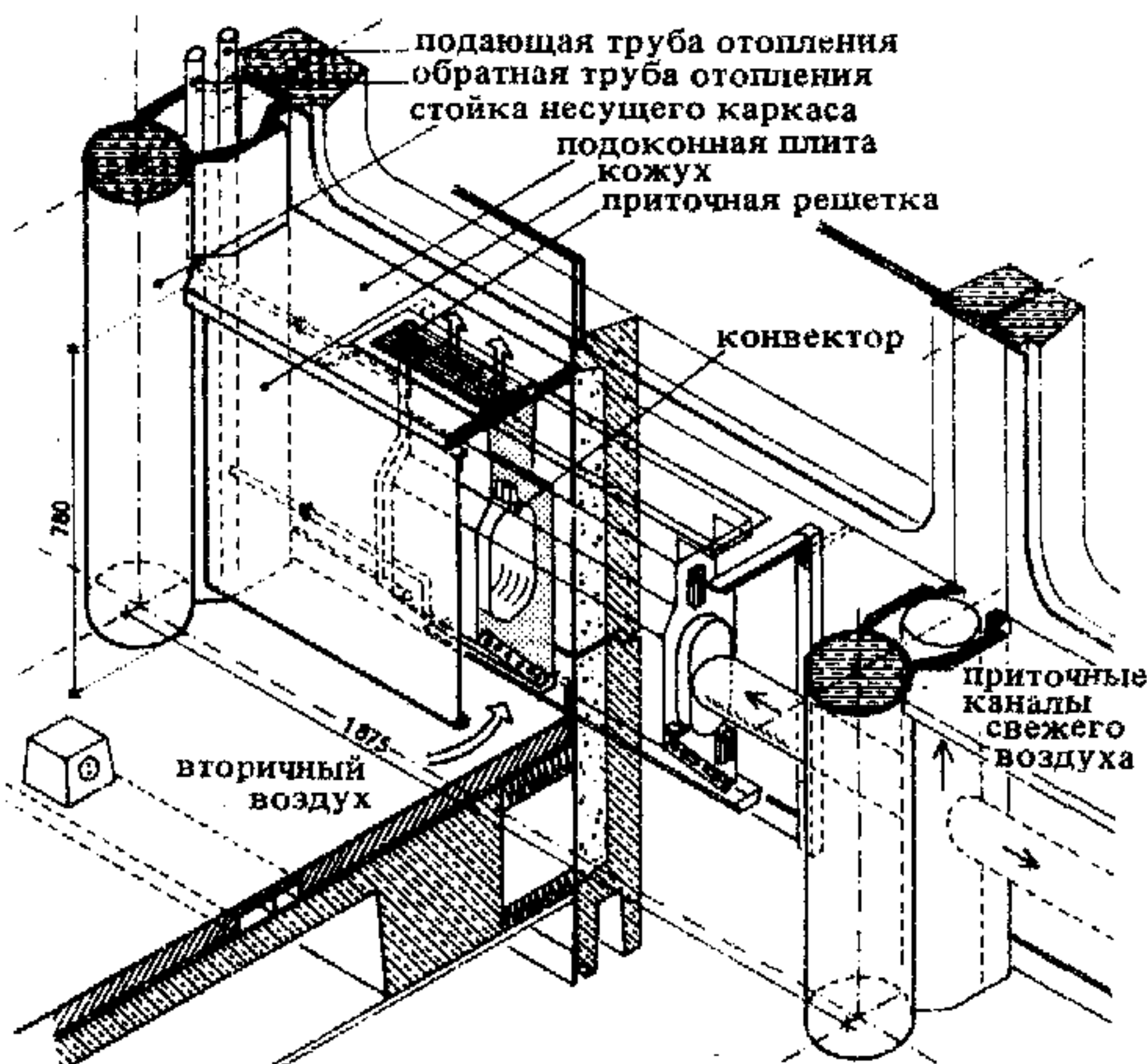
1. Пример высоконпорной системы кондиционирования воздуха (система LTG) — административное здание фирмы «Дикергоф цемент». Архит. Э. Нойферт, 1961 г. (см. с. 250)
