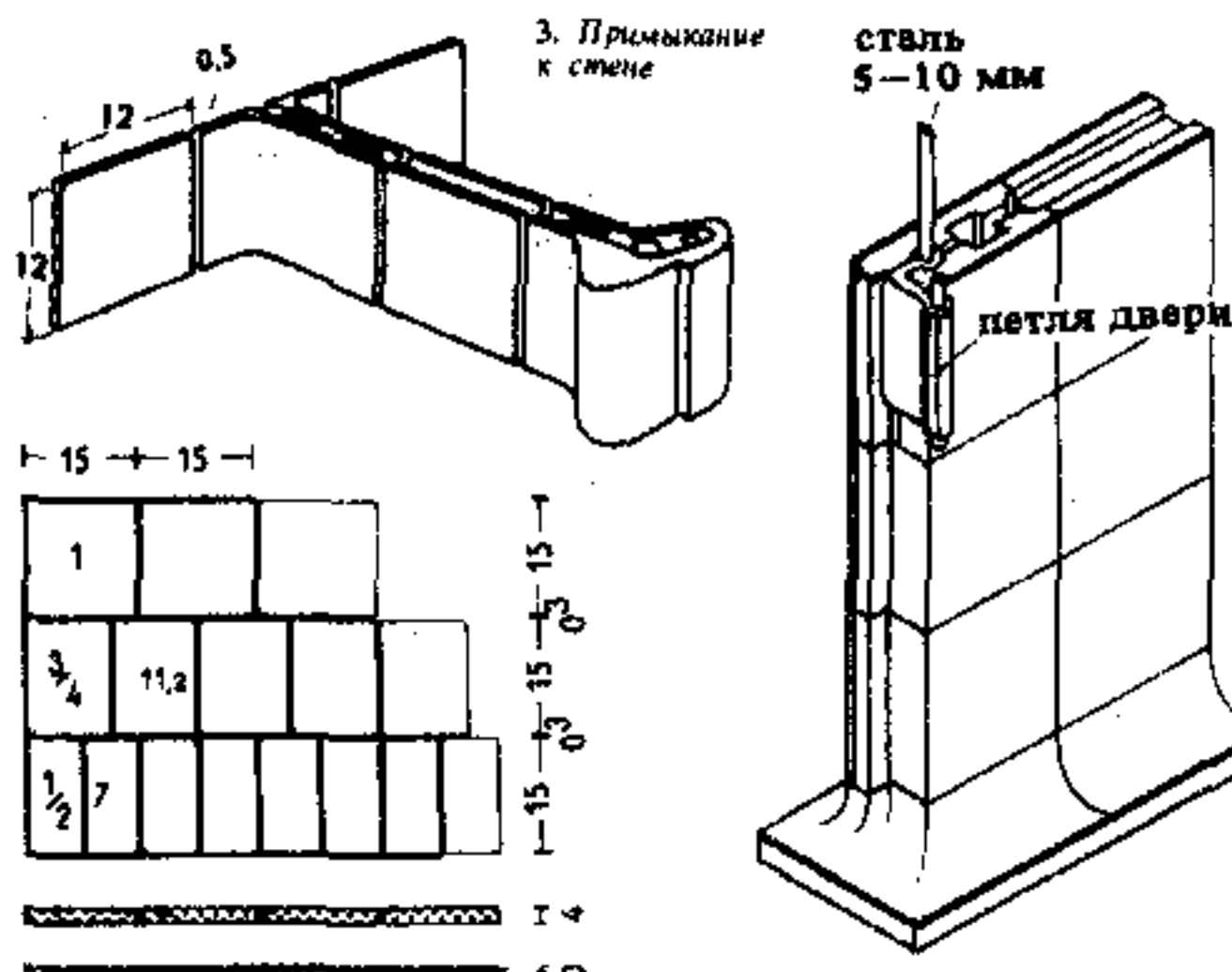
5. Дверная четверть из фасонных элементов
