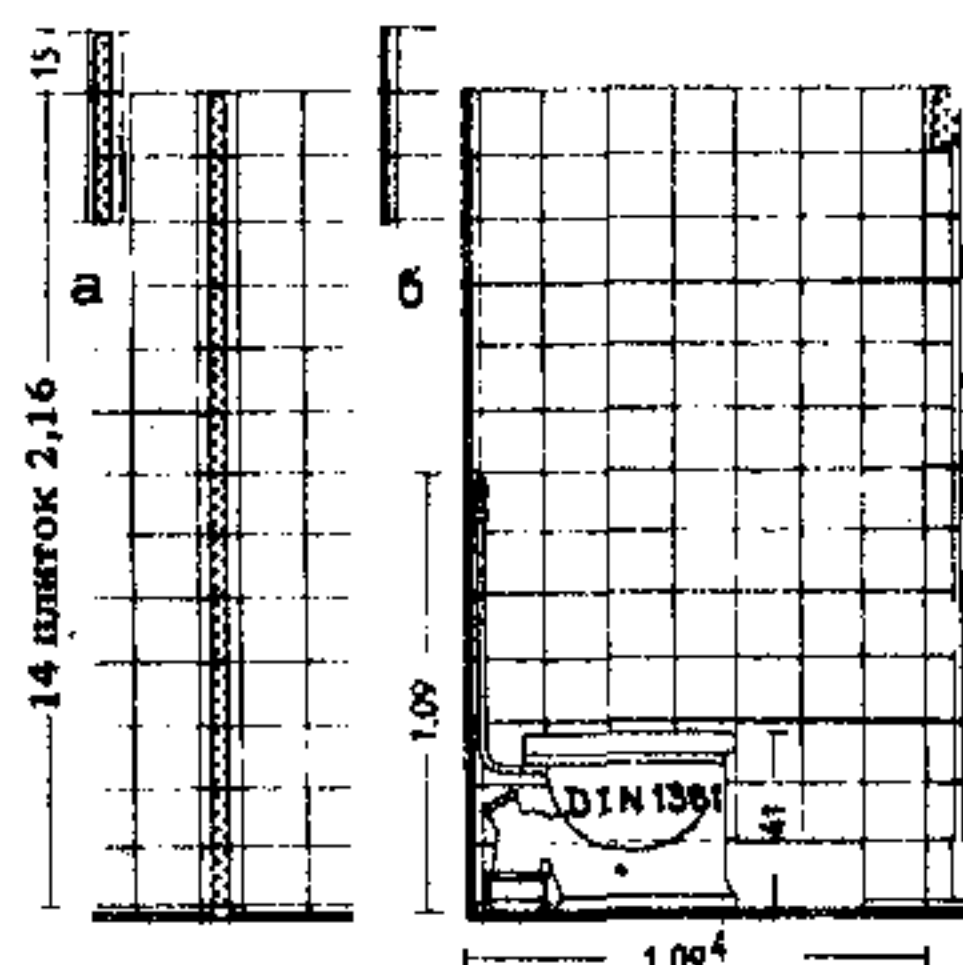
2. Кабина уборкой минимальных размеров
