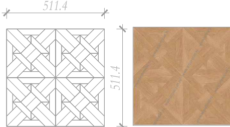
раскладка паркета в пом №:1.08
