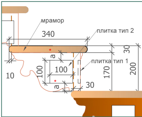
Фрагмент 1. М 1:15
