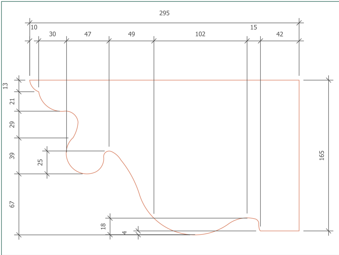
Фрагмент 7 М 1:5
