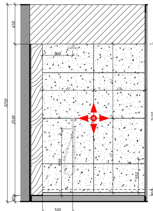
Развёртка 6,4-6,1
