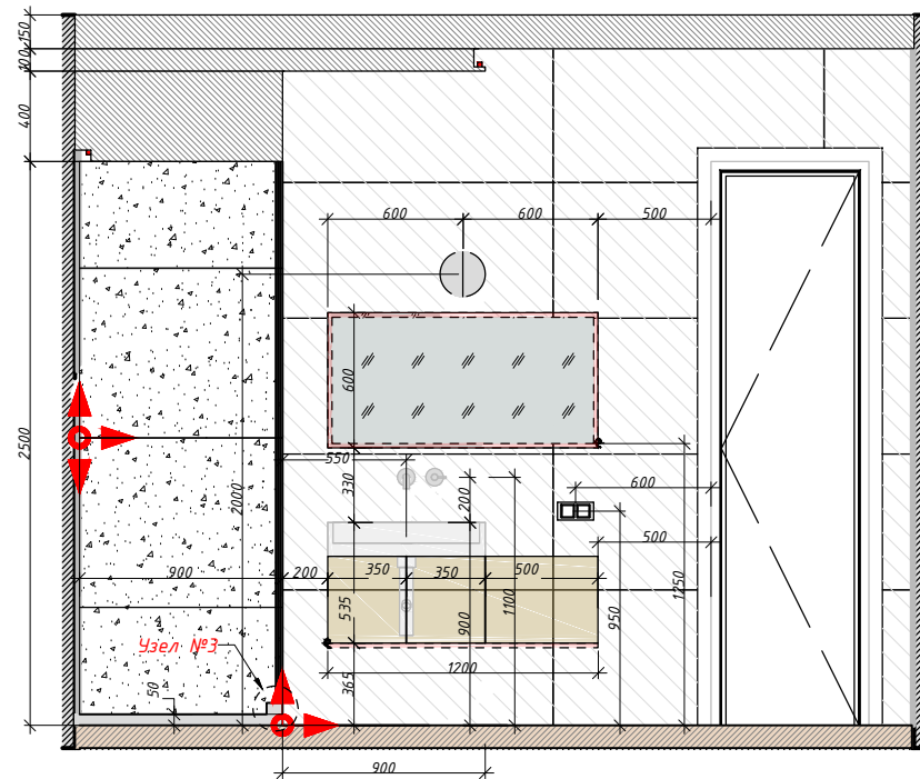
Развёртка 6,3-6,4
