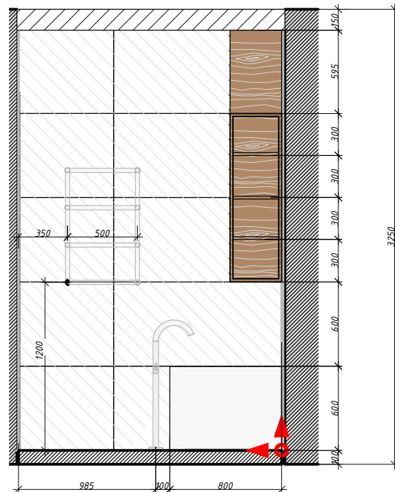
Ограждение душа
