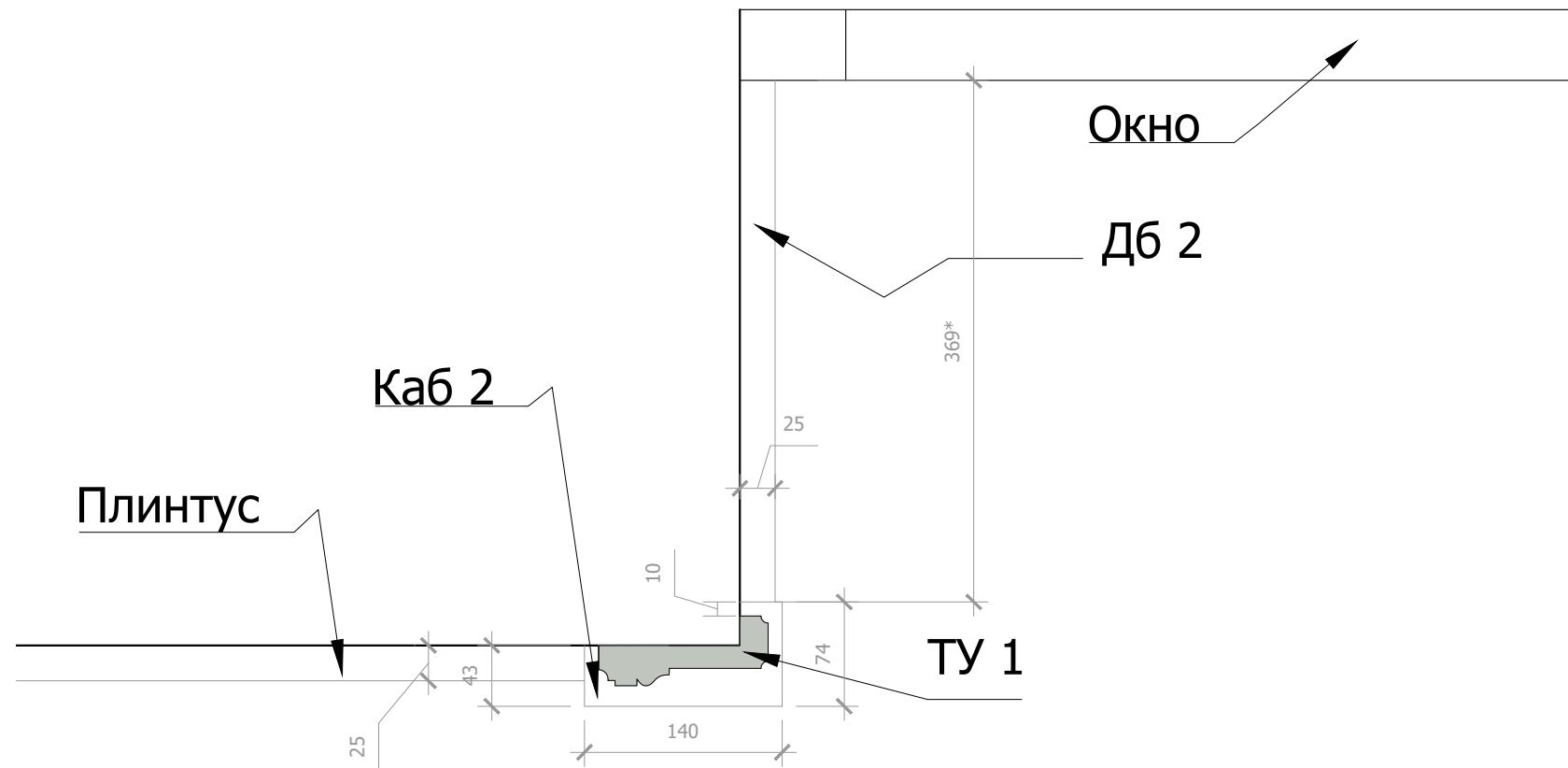
Разрез 1-1. М 1:5
