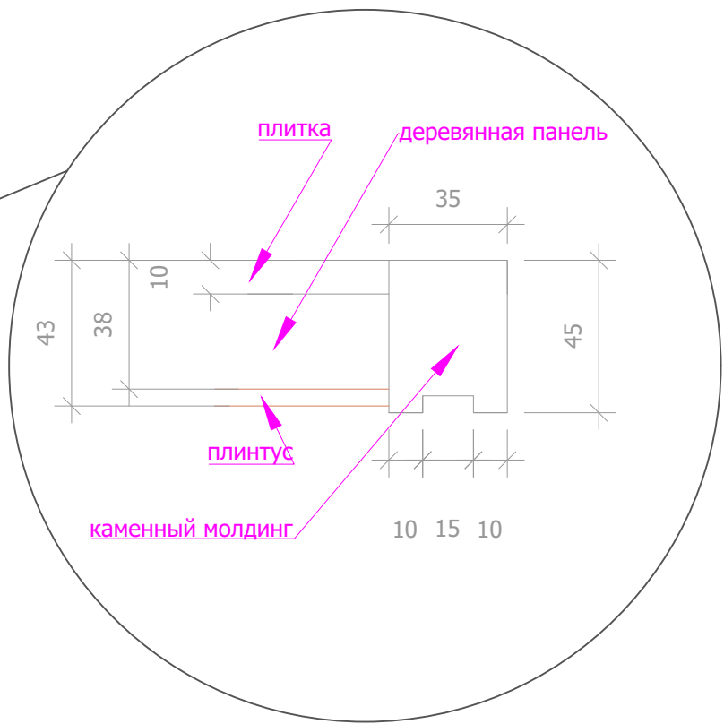
Молдинг-камень. М 1:2
