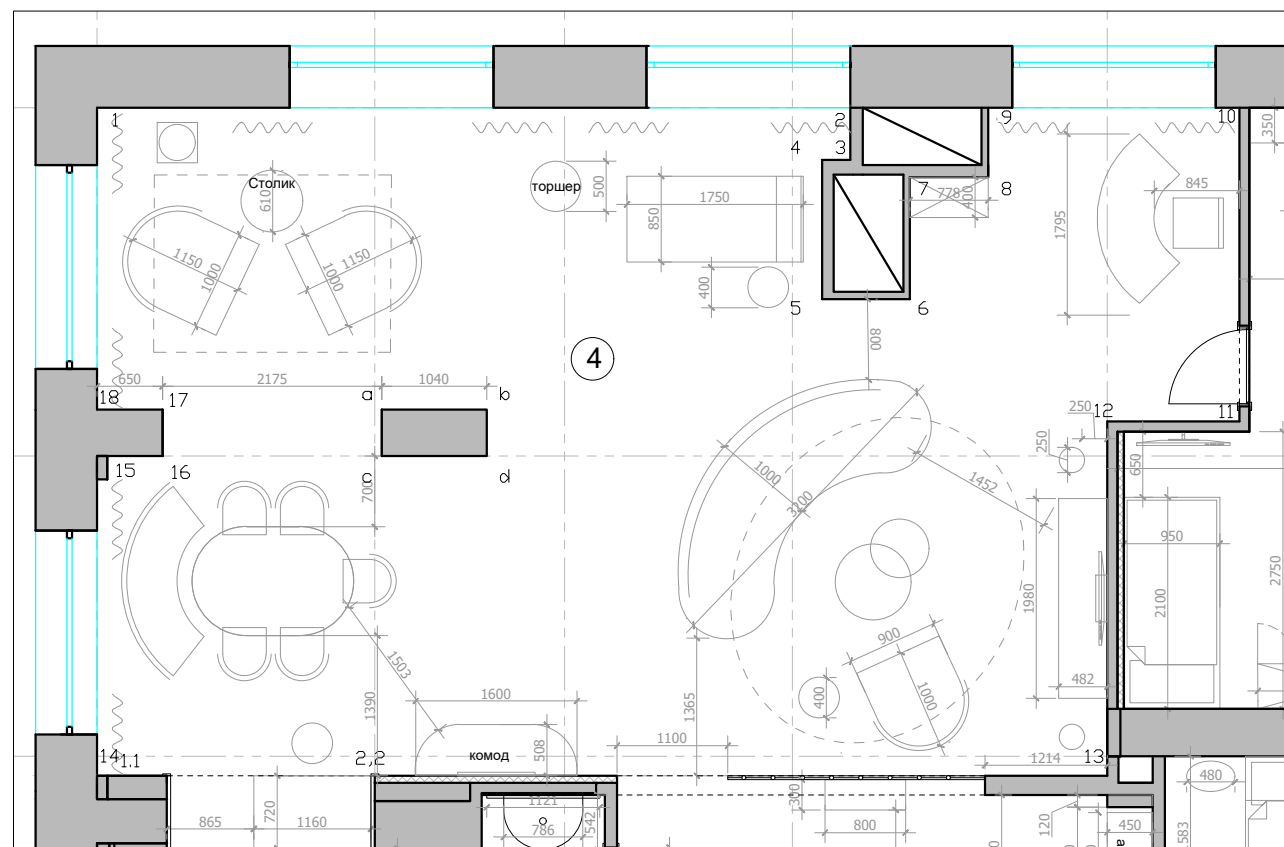
План гостиной 1:75
