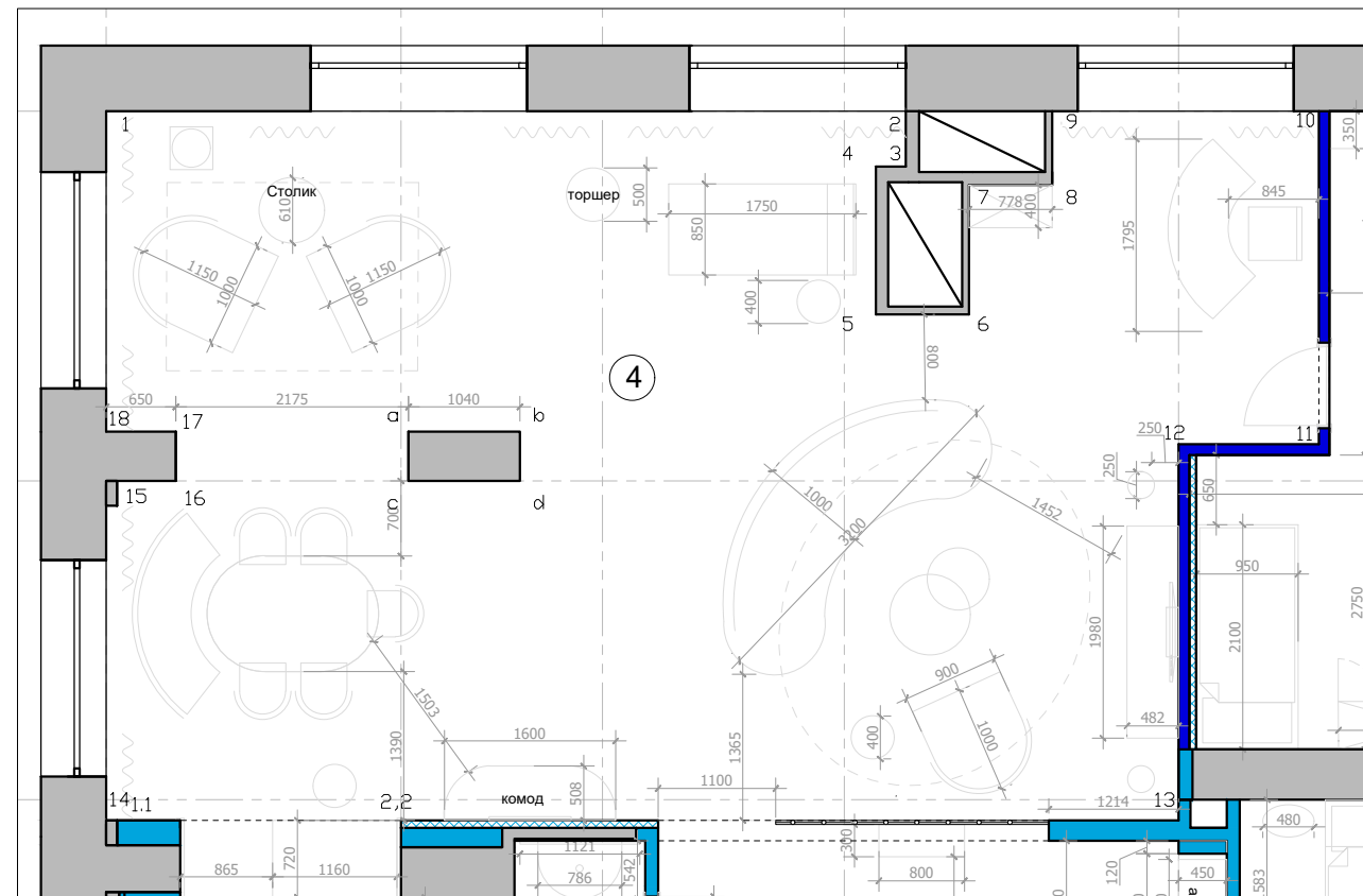
План гостиной 1:75
