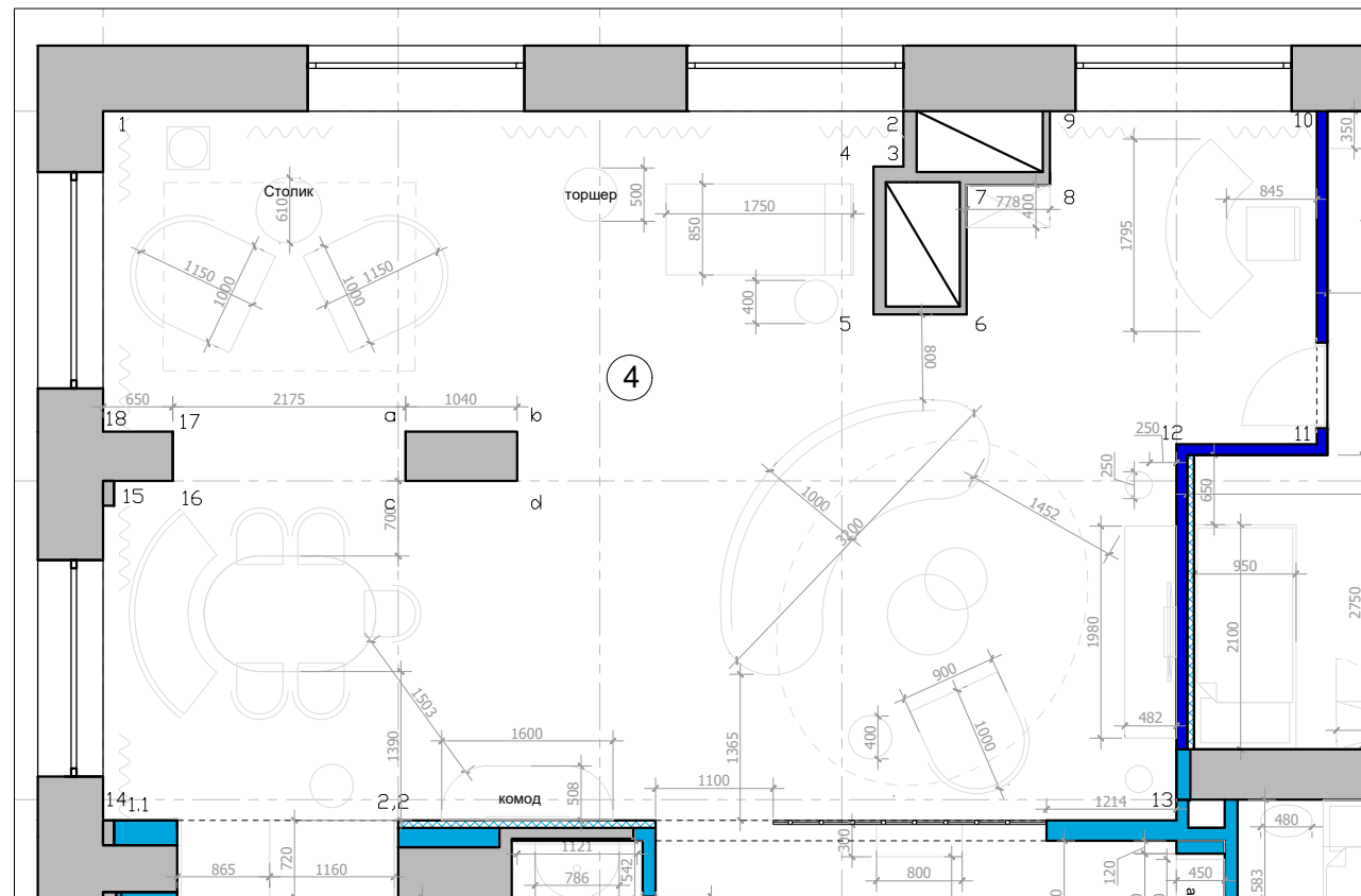
План гостиной 1:75
