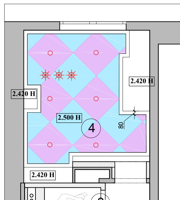
План потолка
