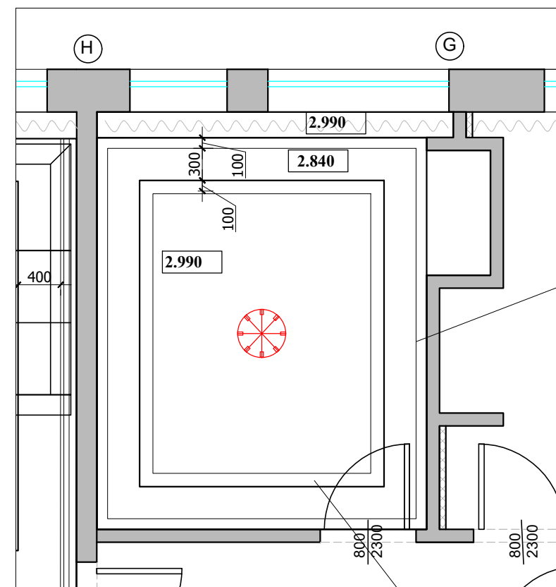
План потолка
