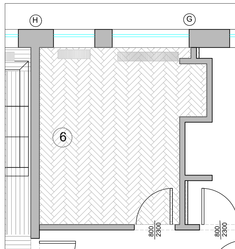
План пола
