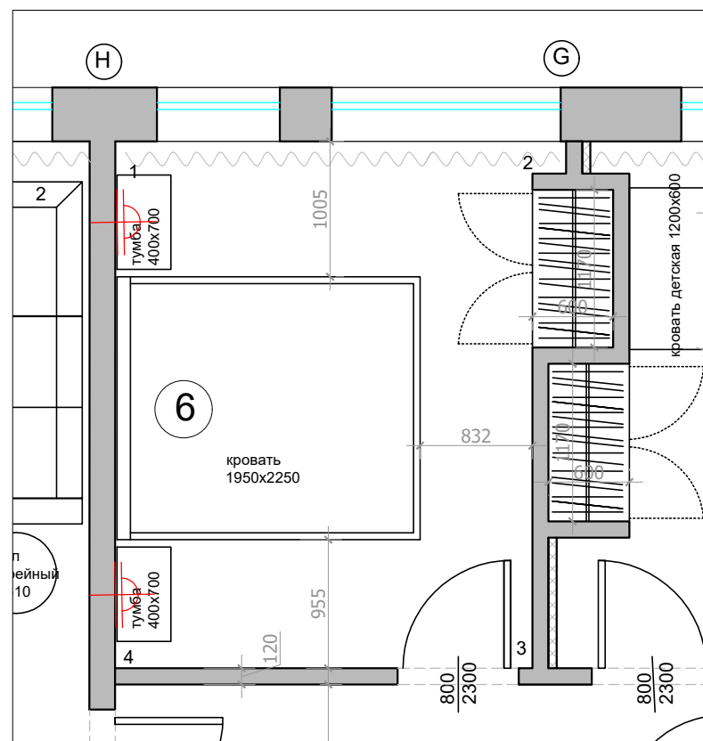
План мебели
