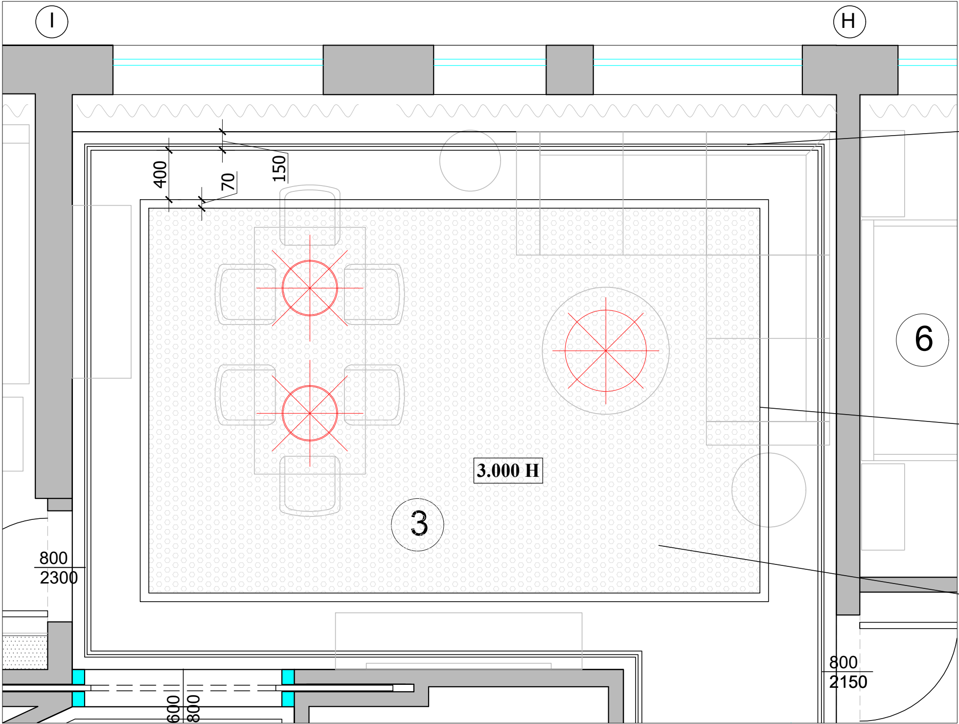
План потолка
