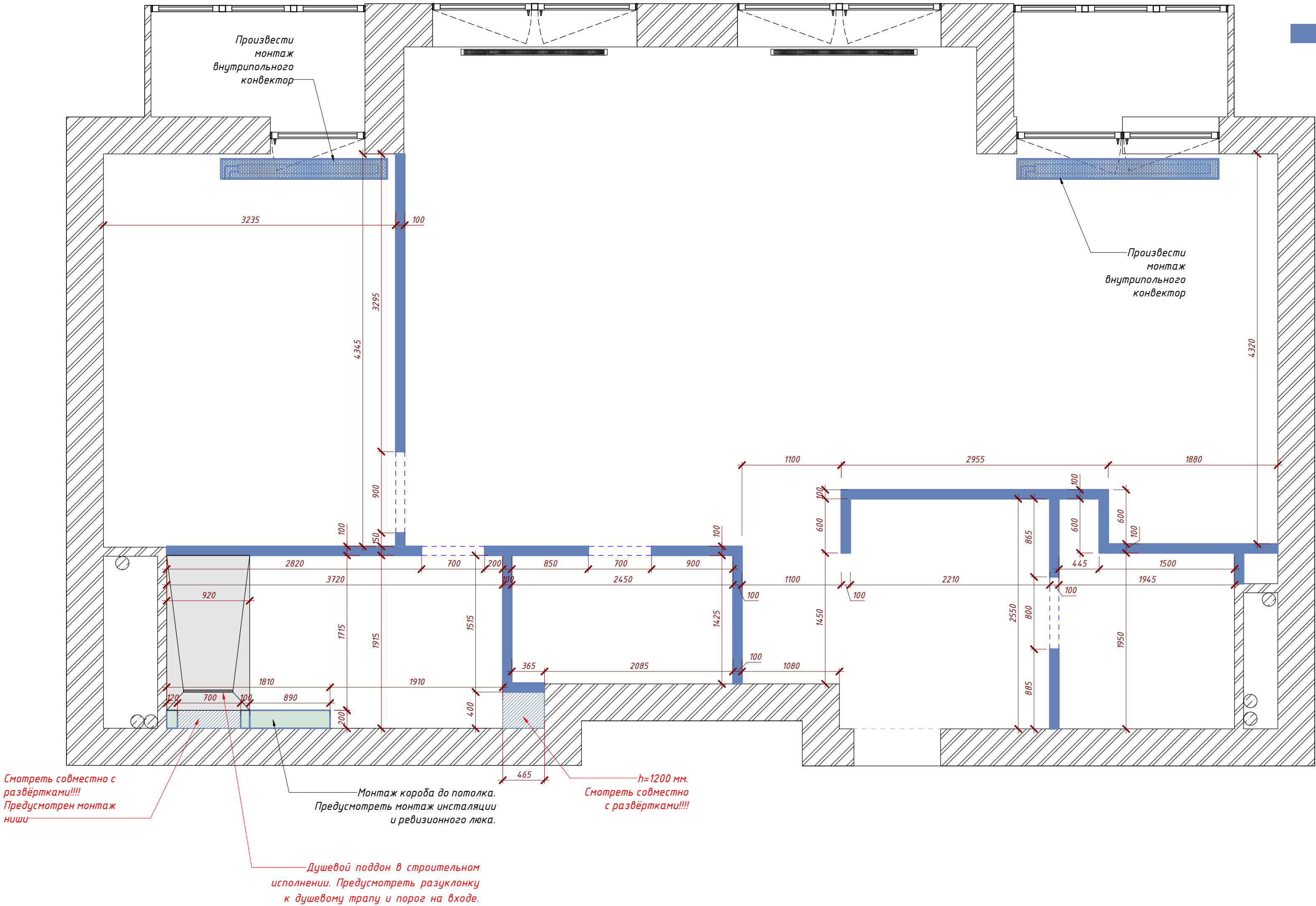
Монтажный план
