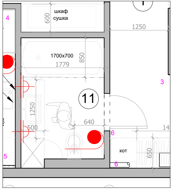
План мебели
