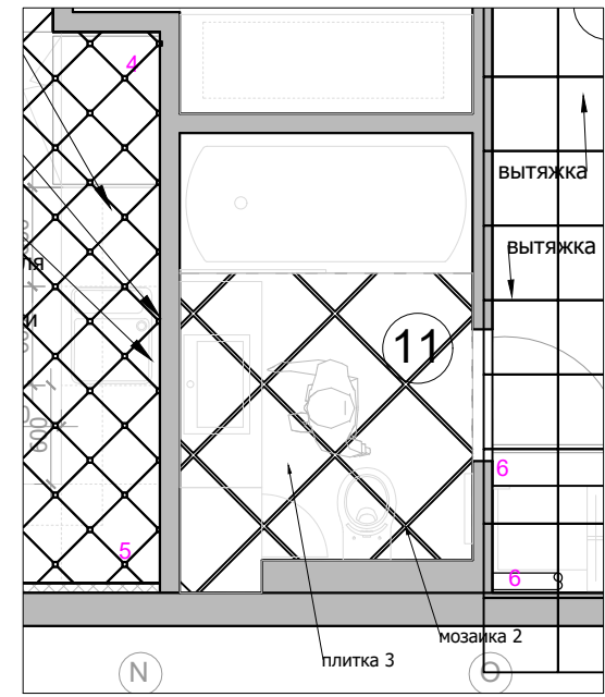
План пола
