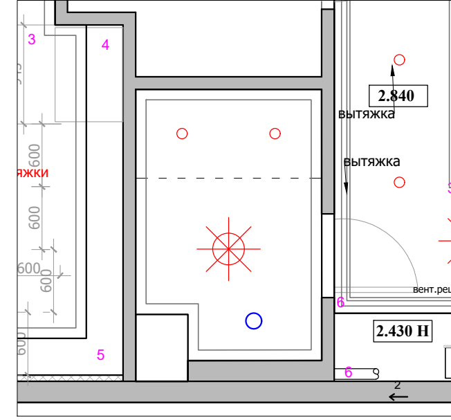
План потолка
