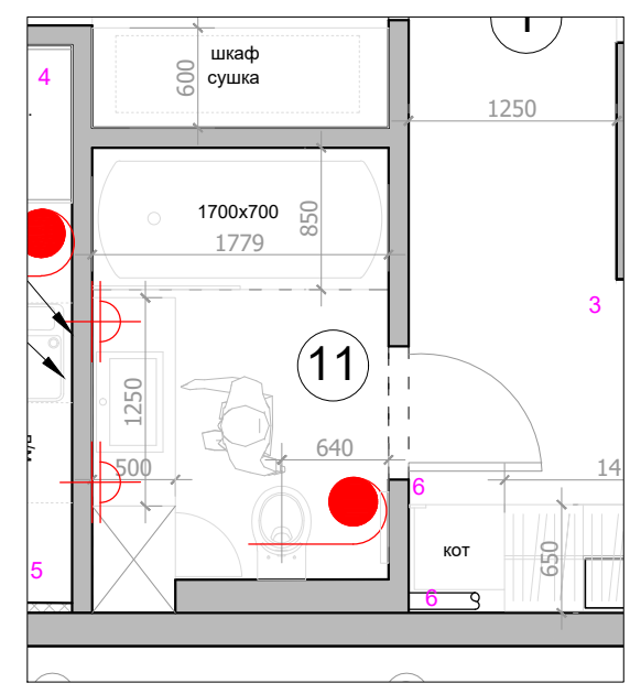
План мебели
