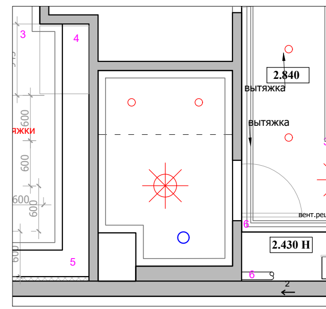
План потолка
