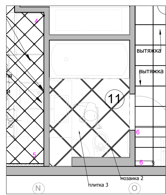
План пола
