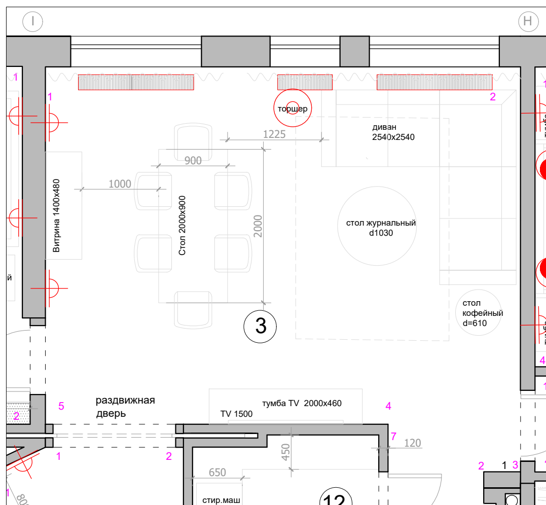
План мебели
