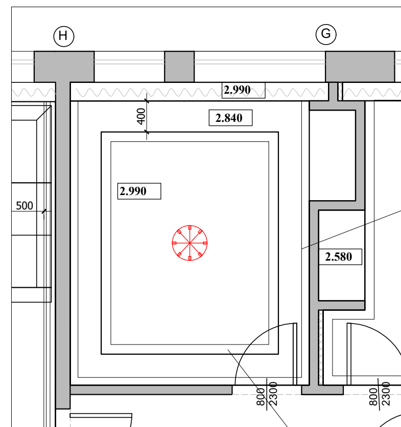
План потолка
