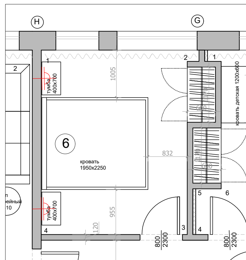
План мебели
