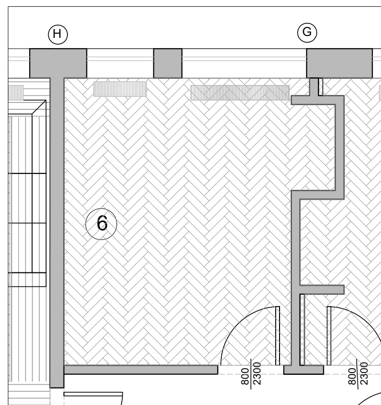
План пола
