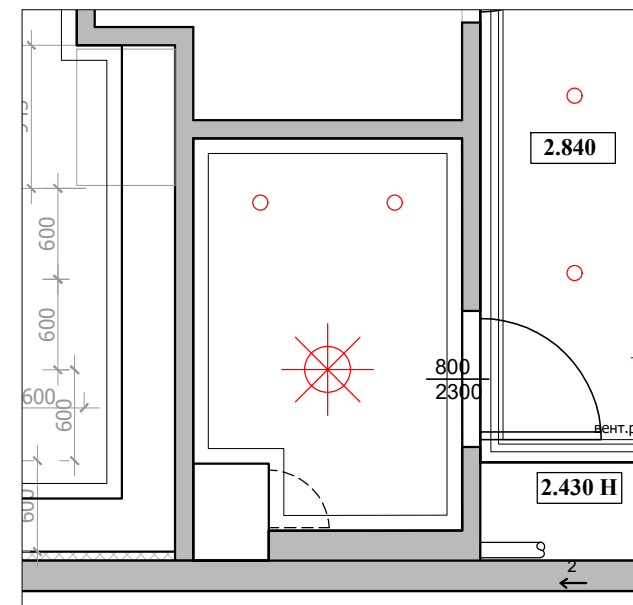
План потолка
