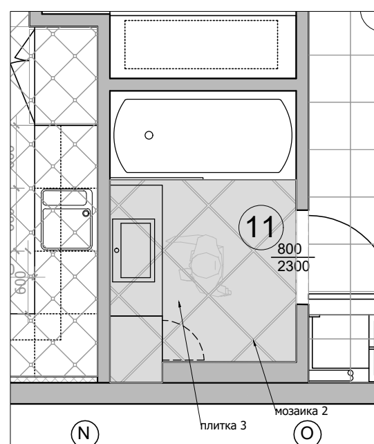
План пола
