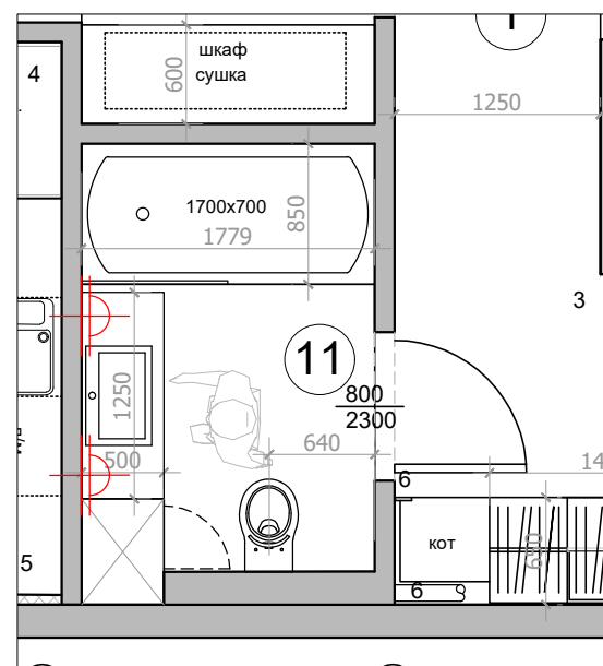
План мебели
