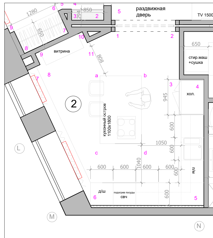
План мебели
