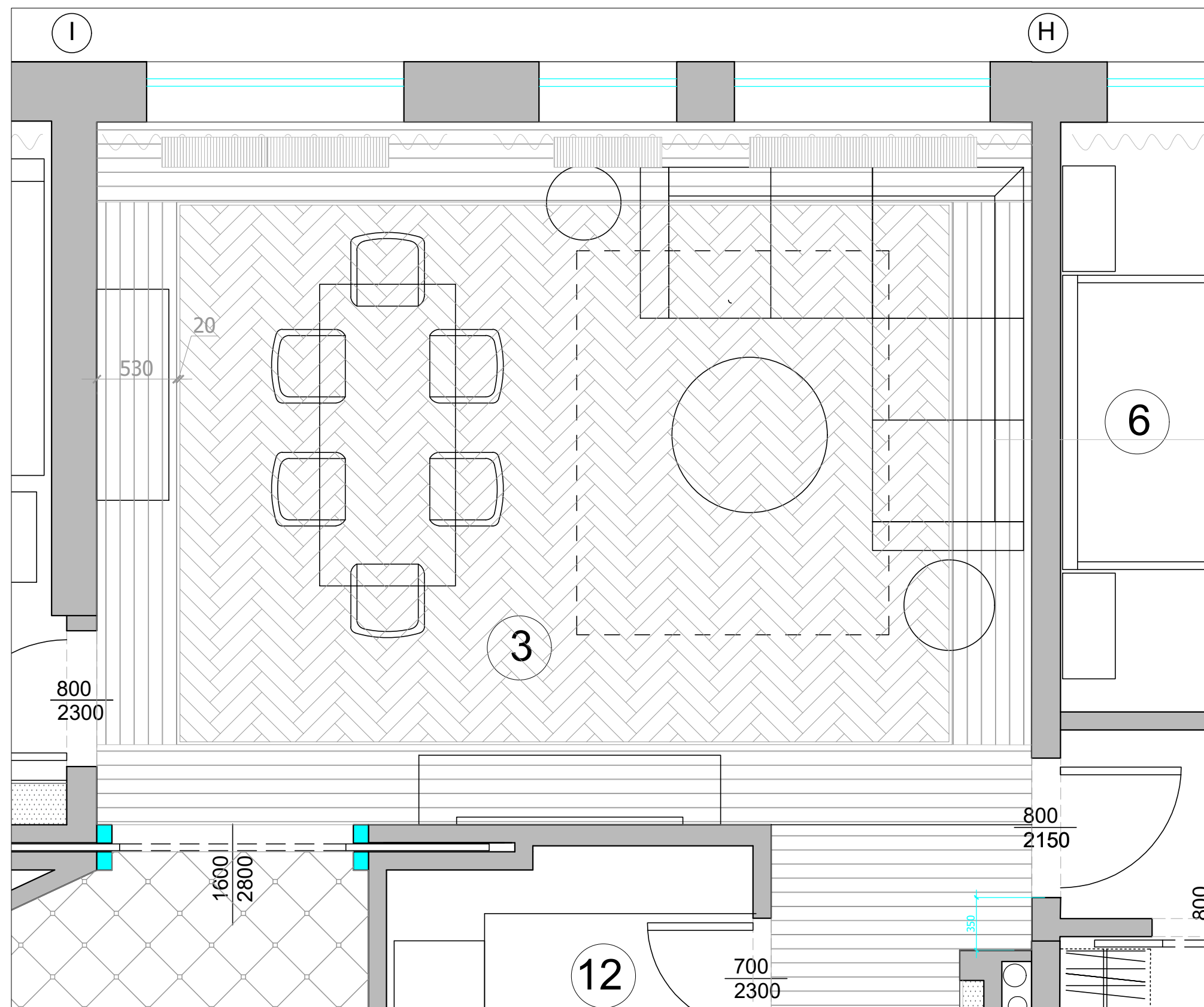
План пола
