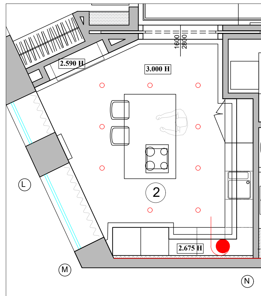
План потолка и светильников
