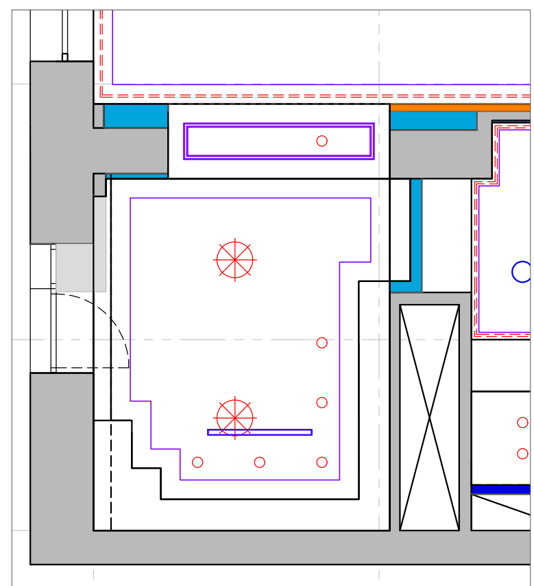
План потолка, света
