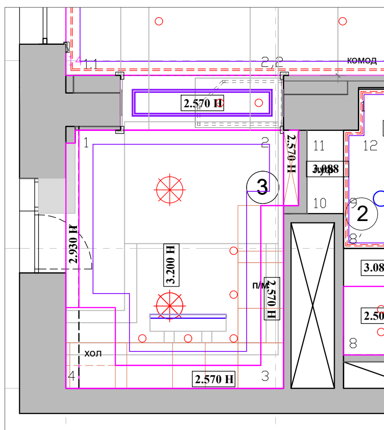
План потолка, вентиляции света
