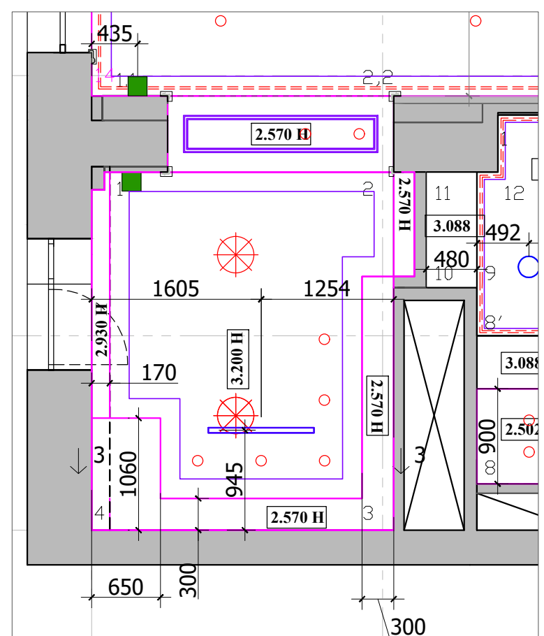
План потолка, света
