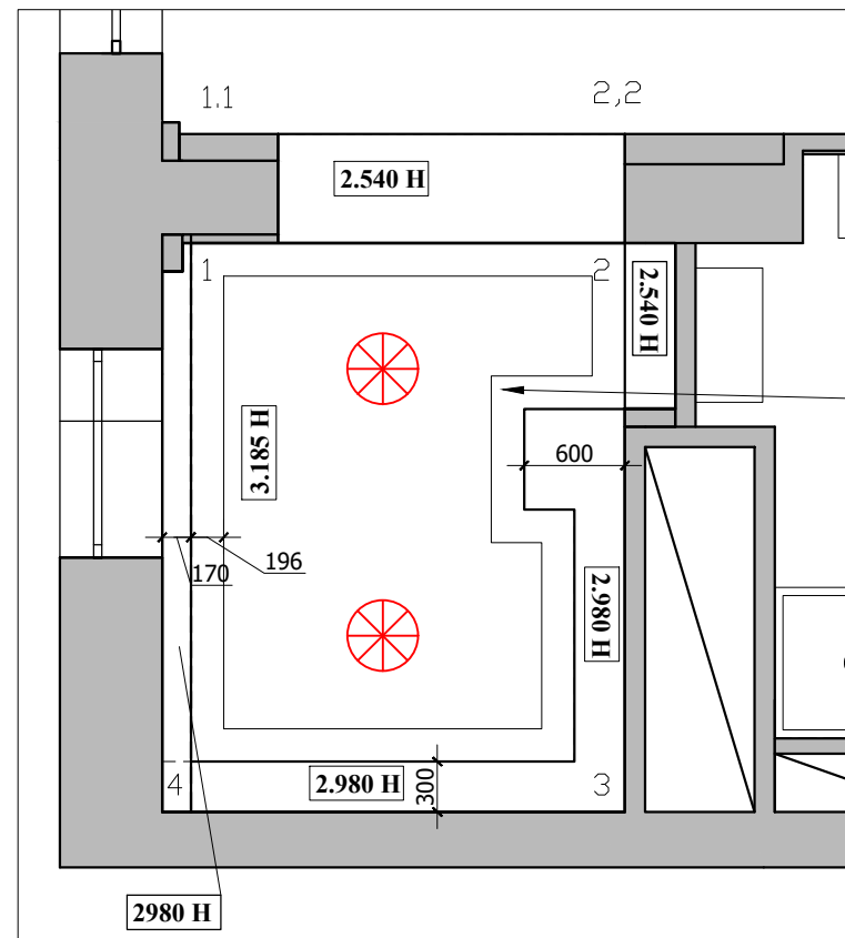
План потолка
