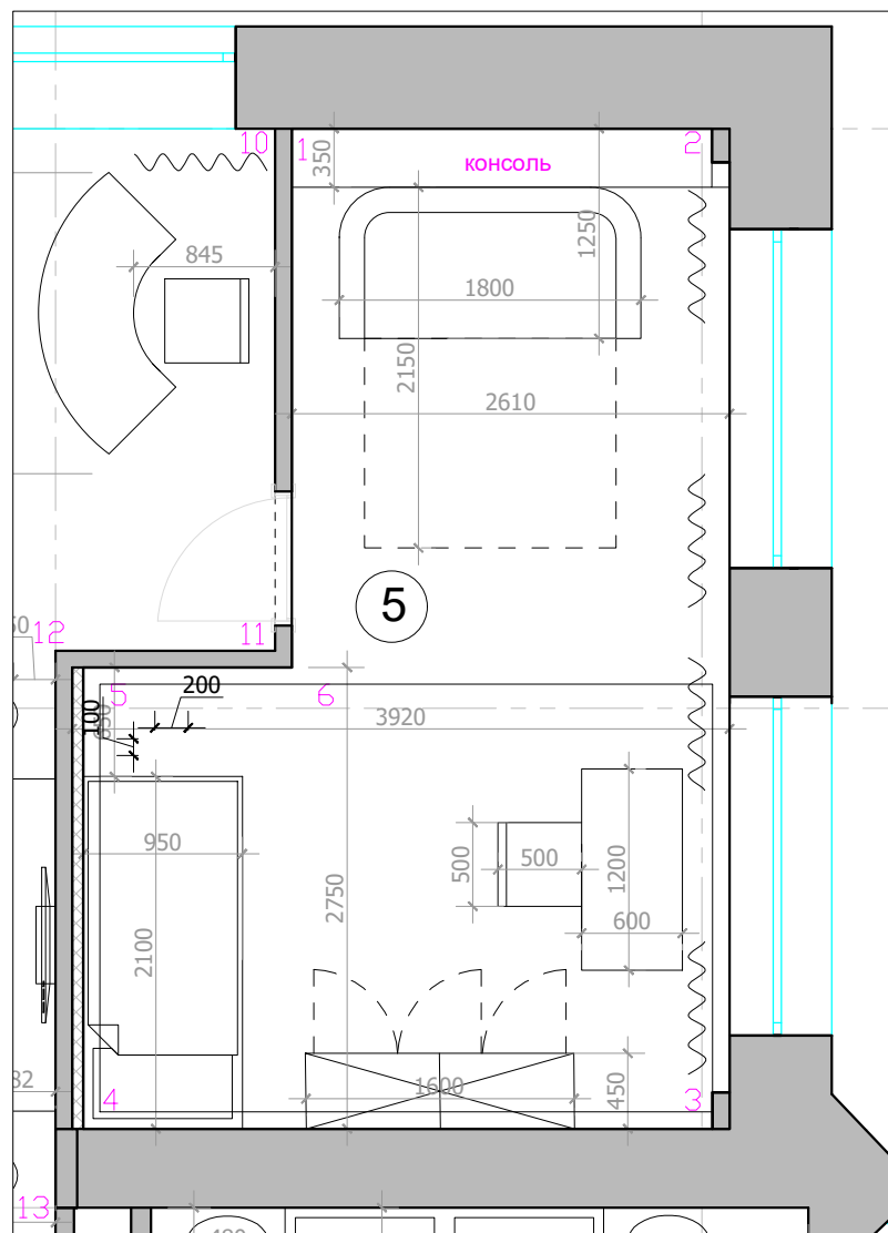
План детская 1:50
