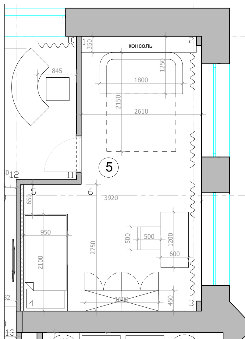
План детская 1:50
