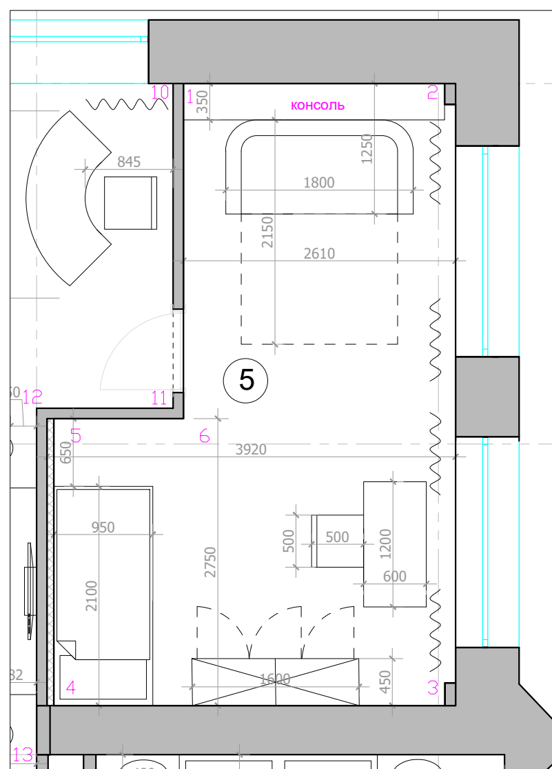
План детская 1:50
