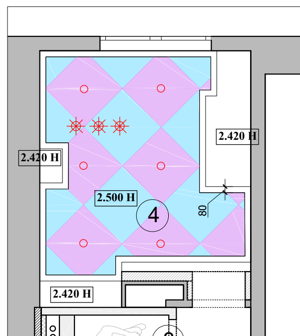
План потолка
