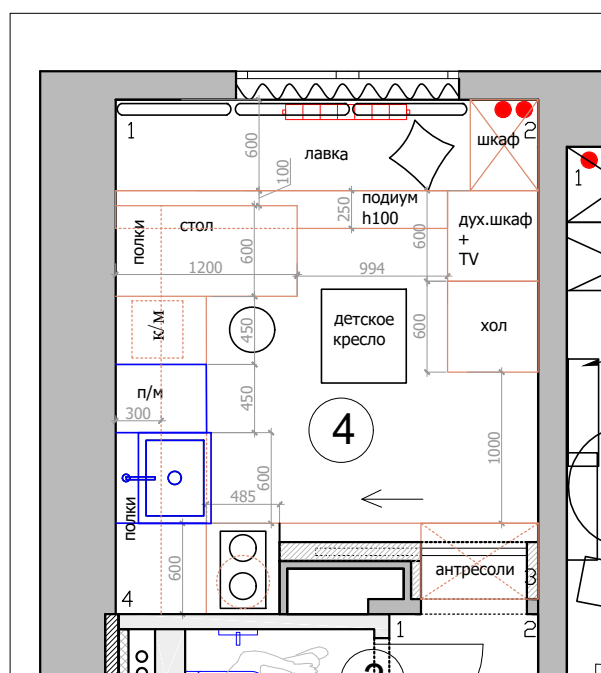
План мебели
